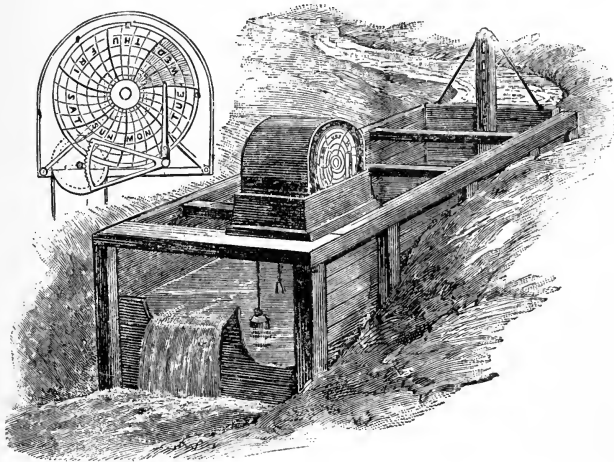
FIG. 44—WATER REGISTER.
