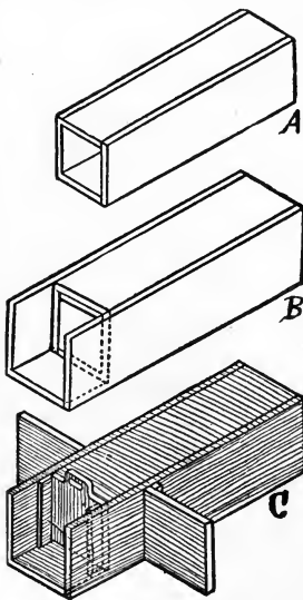
FIG. 99—THE VAN HORN TAP GATE.
