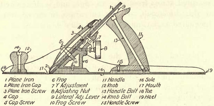
FIG. 145.—PLANE.
