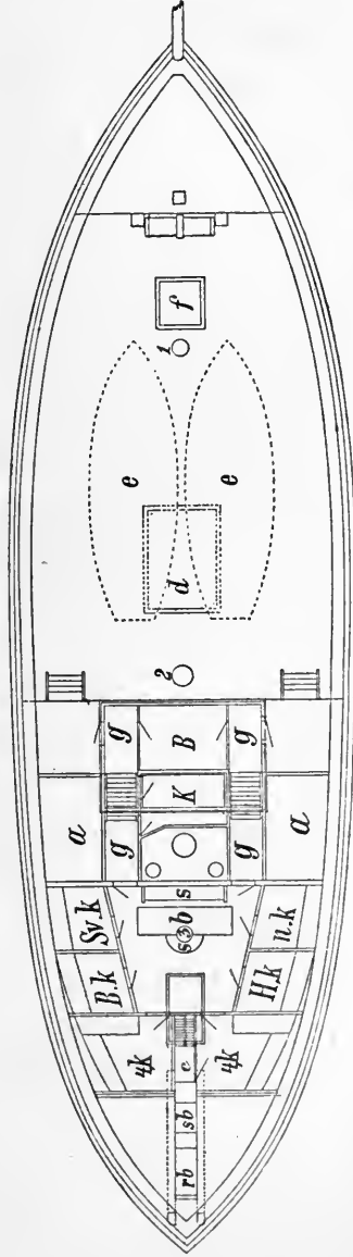
Fig. 2. Plan.
