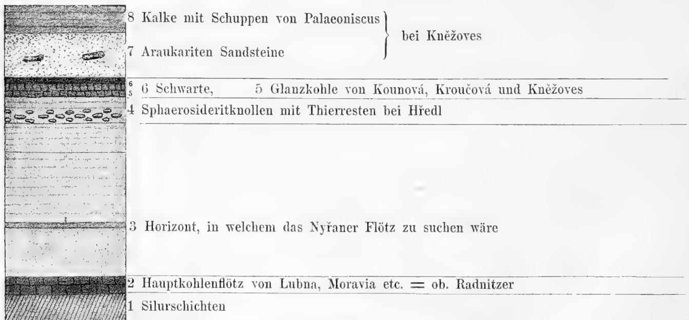
Nro. 13. Schematische Skizze der Schichtenfolge im Rakonitzer Becken.
