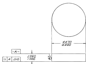
② WINDOW (4 1/2" NOM DIA)
