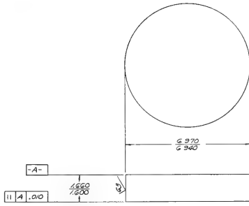
① WINDOW (7" NOM DIA)
