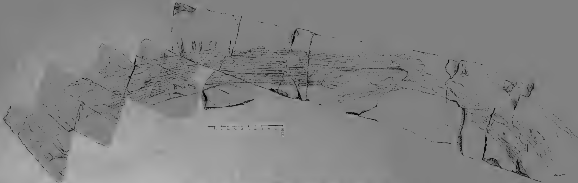
Fig. 65. Pseudosporochnus Krejčii , (Stur ex parte) P. et H.
