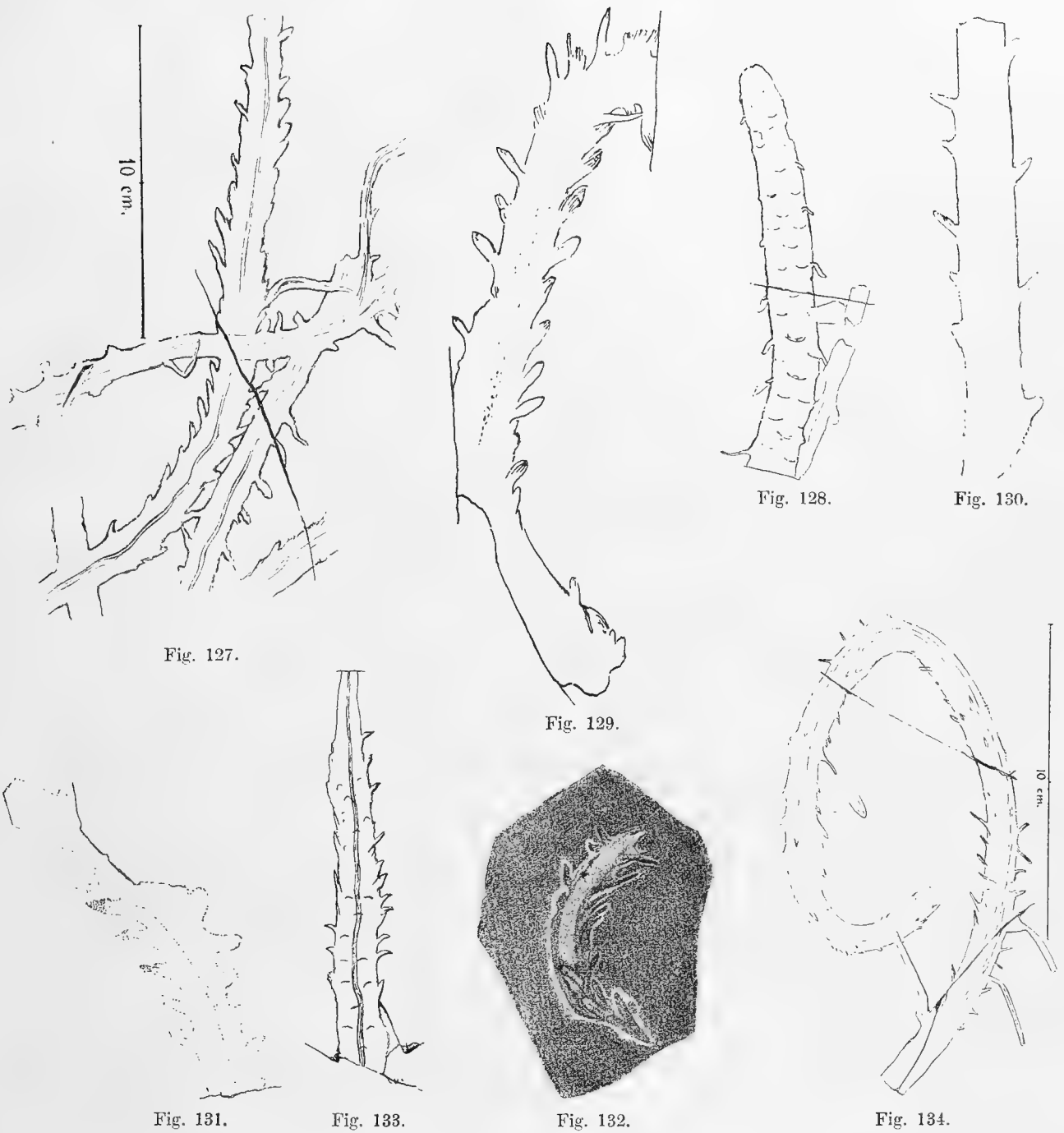
Fig. 127—134. Psilophyton spinosum , (Kr.) P. et B.
