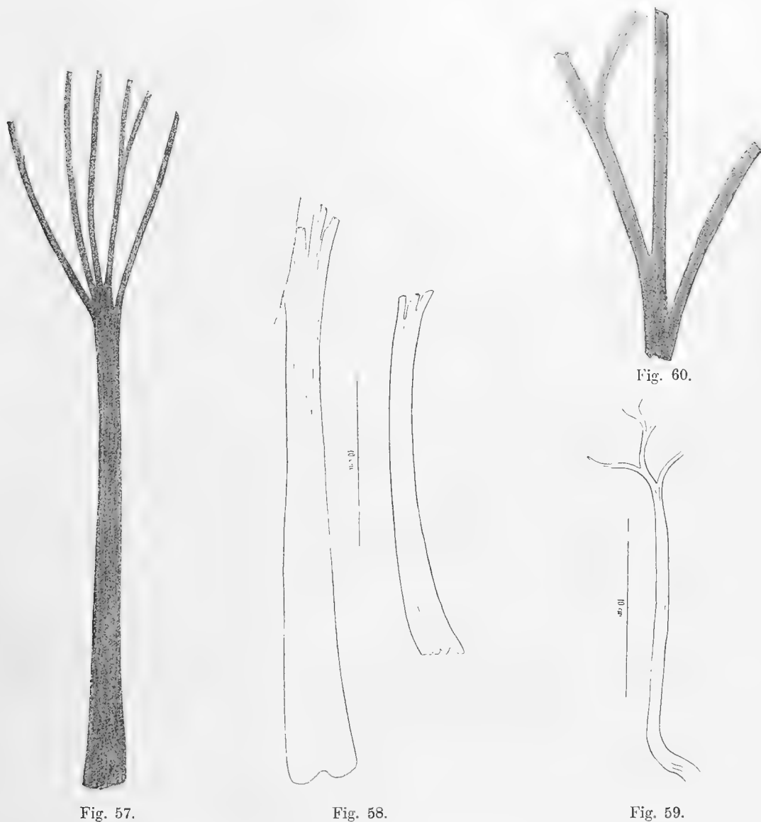
Fig. 57—60. Pseudosporochnus Krejčii , (Stur ex parte) P. et B.
