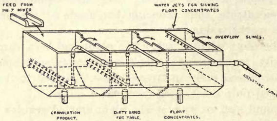
FIG. 21. EXPERIMENTAL SPITZ-BOX.
