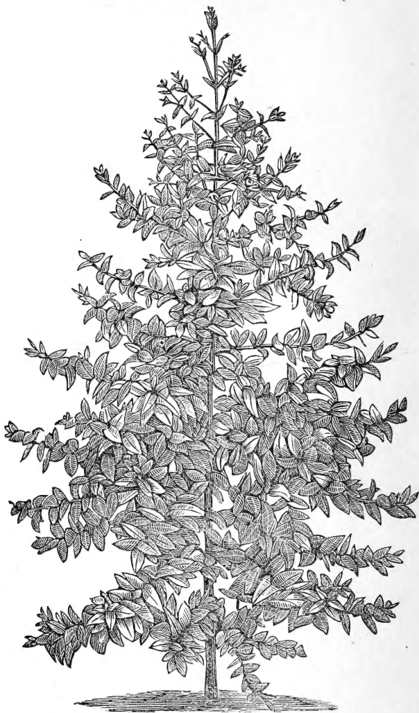
Eucalyptus Globulus.
