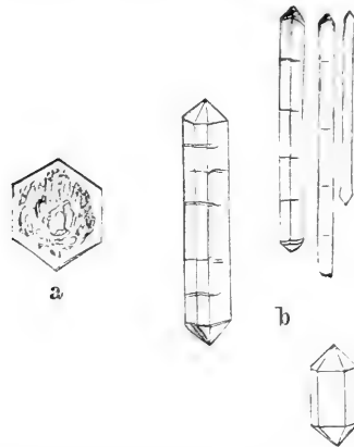
Abb. 20. Mikroskopische Avatitkristalle.
