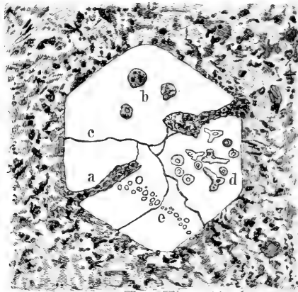
Abb. 15. Zerprungenes Quarzkrystall in Felsitporphyr.
