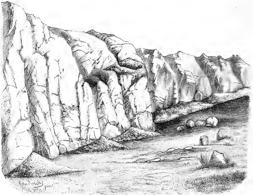
Abb. 17. Trodenener Abtrag der Verwitterungsprodukte.
