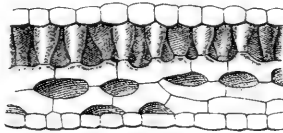
Abb. 24. Theil des Durchschnittes eines im Schatten erwachsenen Buchenblattes (nach Stahl). Die Parenchymischicht des Blattes ist flaschenförmig ausgebildet. (Form fast aller ausgesprochenen Schattenpflanzen.)
