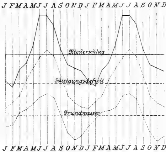
Abb. 1. Doppeljahresperiode des Niederschlags, des Sättigungsdefizits und des Grundwasserstandes in München. (Nach Zopya.)
