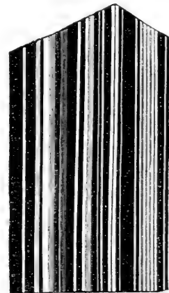
Abb. 19. Durchschnitt eines Plagioklastkrystalles im polarisirten Licht betrachtet. Jede helle oder dunkle Linie entspricht einem Krystallindividuum, die gleichmäßig zu Gesamtkrystallen verwachsen.
