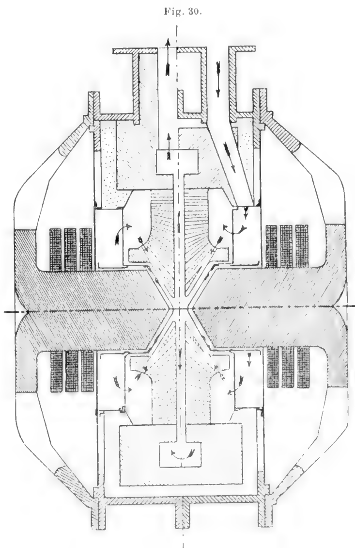
Schematische Darstellung eines neueren Ofens von Birkeland und Eple
