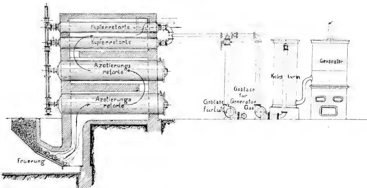
Azotierungsanlage.
