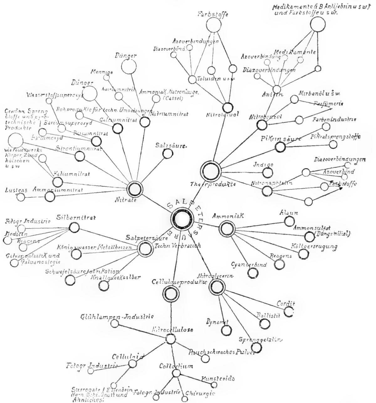
Salpetersäure und ihre Anwendungen in Landwirtschaft und Industrie. Nach Birkeland und Eyde.
