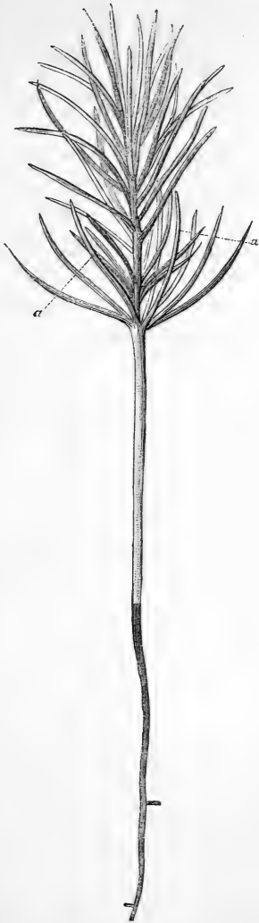
Fig. 1. Spirende Plante af Pinus Laricio . a otte i en Krands stillede Kimblade.
