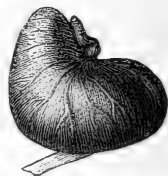
Frugt af Zelkova, lidt forstørret.
