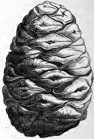
Kogle af Wellingtonia gigantea (nat. Störr.).
