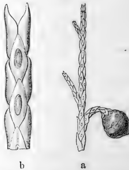
Sabina foetida . a en lille Green. b et Stykke af samme, svagt forstørret.
