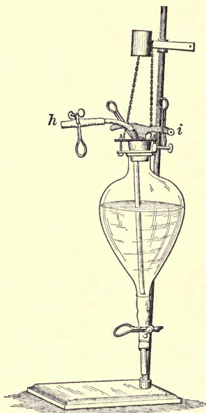
FIG. 2.—SAMPLING APPARATUS.
