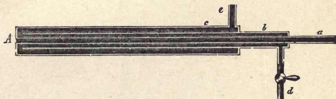
FIG. 1.—GAS-SAMPLING TUBE.
