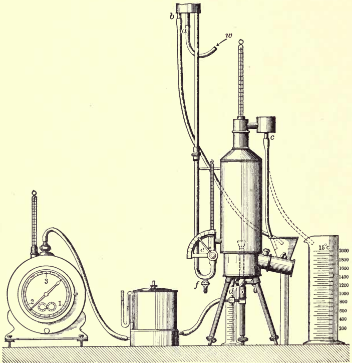
FIG. 20.—JUNKERS GAS-CALORIMETER.
