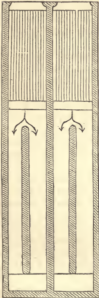
Fig. 95.—Split Draught.
