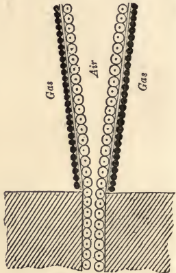
Fig. 15.—Diffusion-jet.
