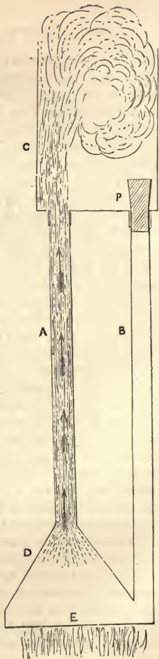
Fig. 73.—Ebullition.
