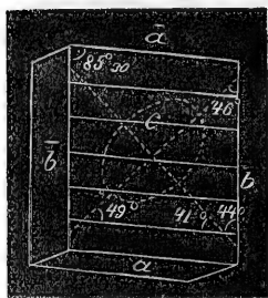
mätta pimelinsyrekrystallerna:
