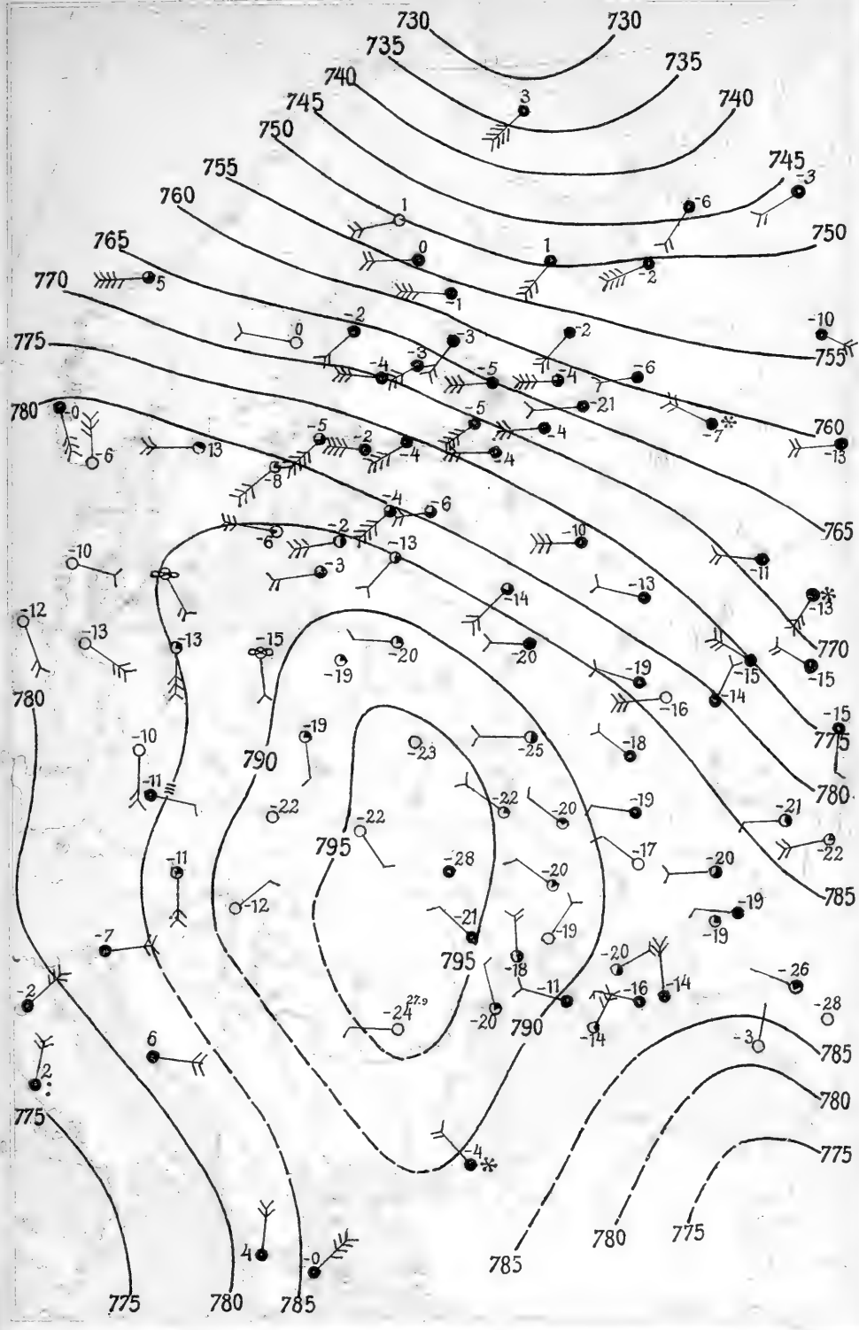
Väderlekscarta för d. 24 jan. 1907 kl. 7 f. m.
