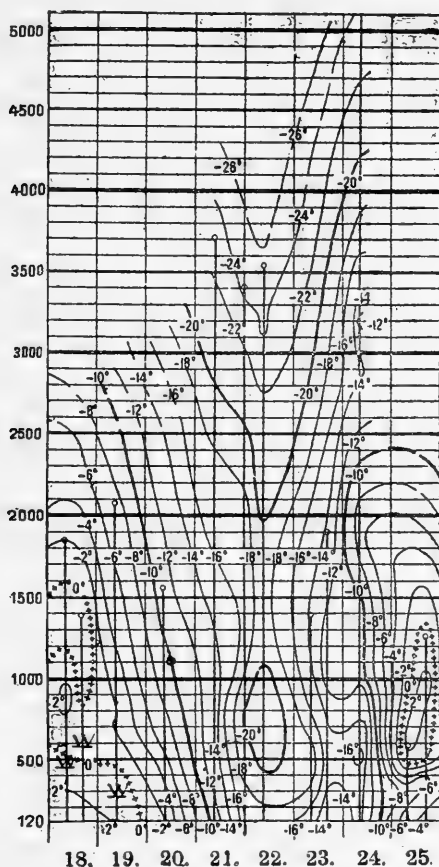
Termoisepleter, åskådliggörande temperaturrens förändring med höjden under dagarna den 18–25 januari öfver Lindenberg nära Berlin.
