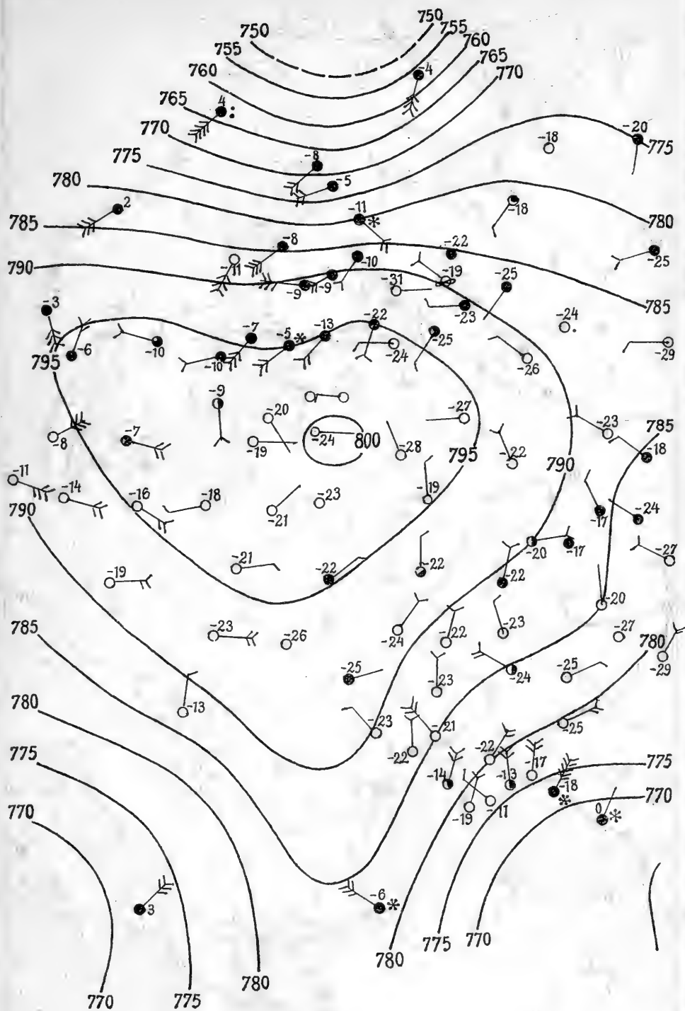
Väderlekskarta för d. 23 jan. 1907 kl. 7 f. m.
