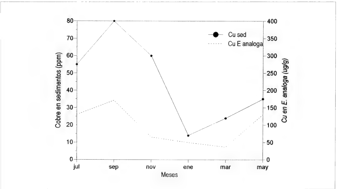
FIGURA 5. Contenido de cobre en sedimentos y en Emerita analoga ( \text{mg/g} , peso seco) de Playa Rinconada. Antofagasta, 1993-1994.
