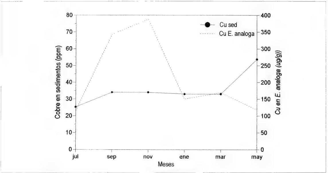
FIGURA 4. Contenido de cobre en sedimentos y en Emerita analoga ( \mu\text{g/g} , peso seco) de Playa Amarilla. Antofagasta, 1993-1994.
