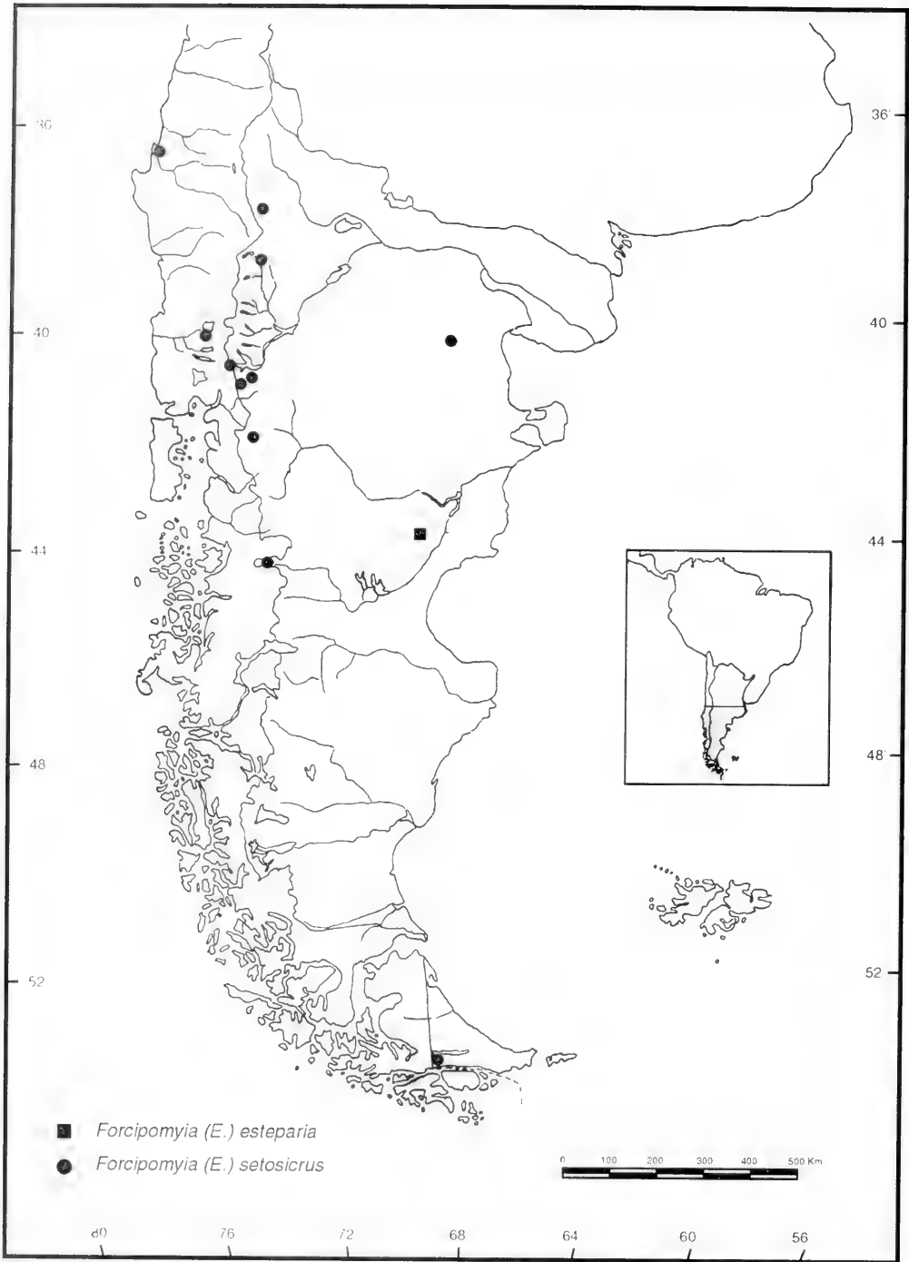
FIGURA 21. Distribución de las especies Forcipomyia (E.) esteparia n. sp. y Forcipomyia (E.) setosicus (Kieffer).
