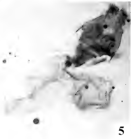
FIG. 1. Lieu de récolte. Sector La Mina. 960 m, Province del Maule, VII Région, Chile. FIG. 2-5. Copitarsia murina n. sp.: 2. adulte du mâle; Armure génitale: 3. valves et 4. aedeagus; 5. armure génitale de la femelle.
