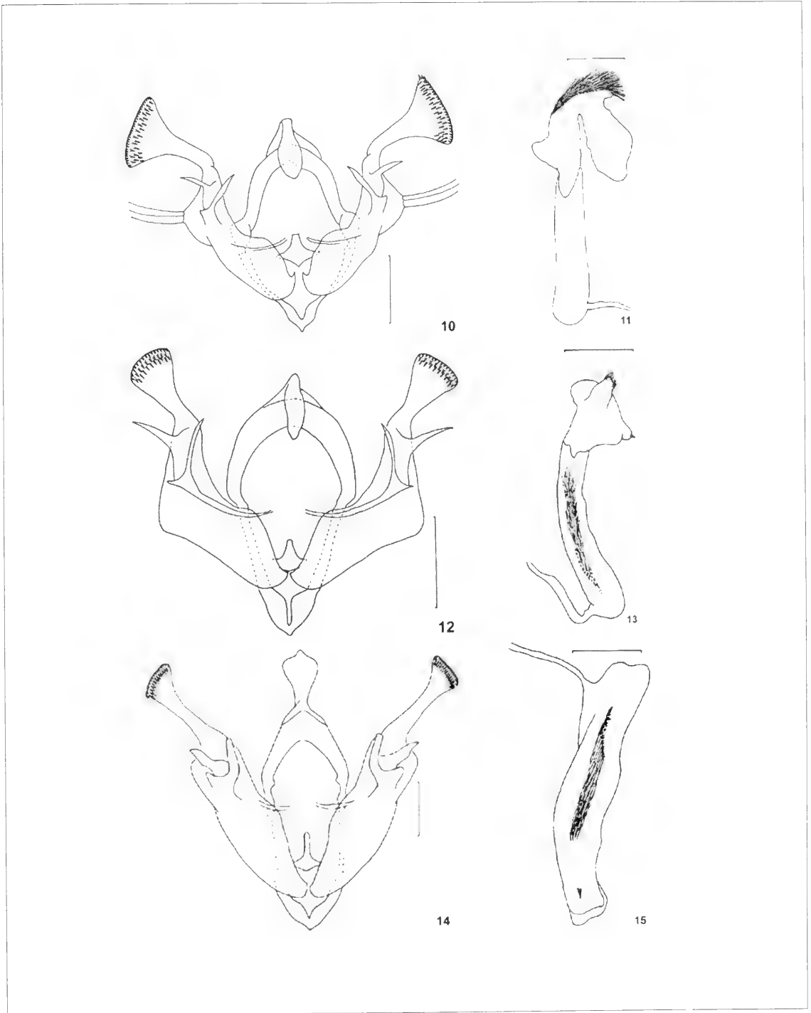
FIGURAS 10-15. Genitalia de los machos. Scriptania maulina n. sp.: 10. Valvas y 11. Aedeago. Scriptania rubroides n. sp.: 12. Valvas y 13. Aedeago. Scriptania viridipennis n. sp.: 14. Valvas y 15. Aedeago.
