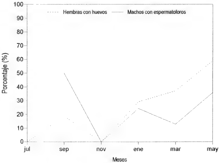
FIGURA 13. Variación temporal del porcentaje de hembras con huevos y de machos con espermatoforos de E. analoga de Playa Rinconada. Antofagasta, 1993-1994.
