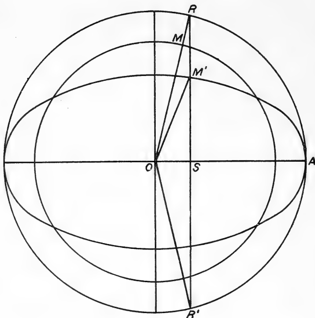
FIG. 44.—Tissot's indicatrix.
