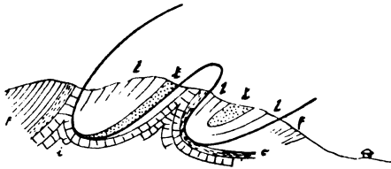
nach Lugeon und Jaccard 1902.
