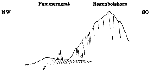
Fig. 10. d Dogger, i oberer Jura, F Flysch.
