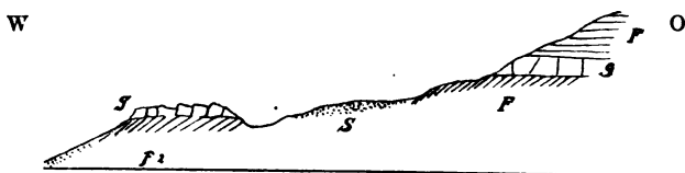
Fig. 9. Alp Sedel. g Gips, F Flysch, S Schutt.
