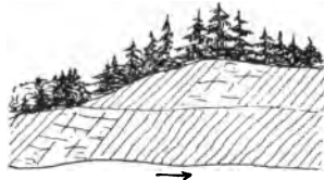
Fig. 16. Zwei Meter weite horizontale Verschiebung im Jurakalk des Laubhornes auf der Westseite des Strässleins unterhalb Rätzliberg.
