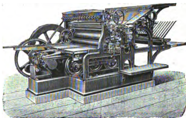
Macchina Tipografica Celere con due rullatori (costruzione usuale)
