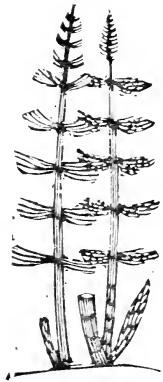
CALAMITES.
