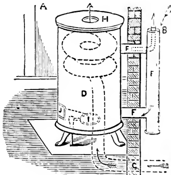
FIG. 14.—GEORGE'S CALORIGEN.
