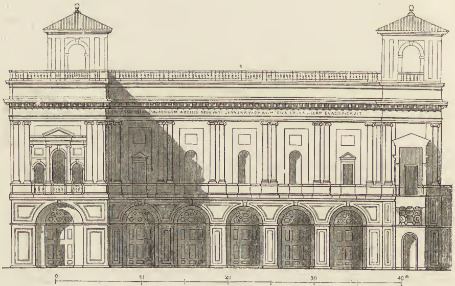
Fig. 209. Monte Imperiale bei Pesaro.
