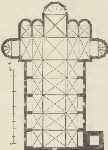
Fig. 116. Servi zu Siena. Grundriss. (L.)
