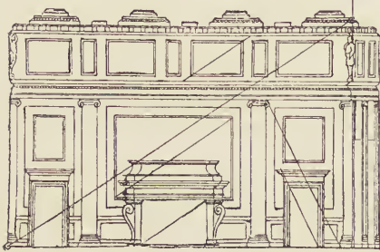
Fig. 64. Hauptsaal des Pal. Massimo in Rom. (Nach A. Thiersch in Durm, Handb. d. Archit.)
