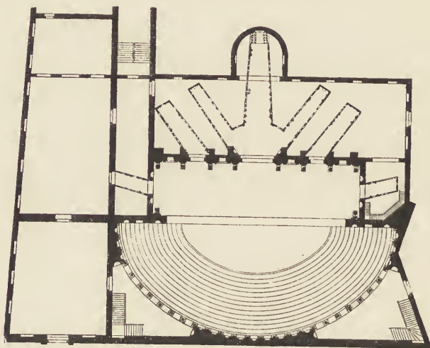
Fig. 282. Palladio's Teatro olimpico zu Vicenza. Grundriss. (Nach Gurlitt.)
