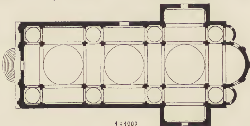
Fig. 138 und 139. S. Salvatore zu Venedig.
