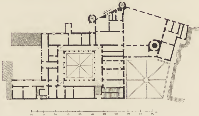
Fig. 164. Palast von Urbino. Grundriss.
