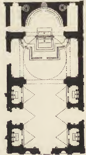
Fig. 127. S. Maria de' Monti. (Nach Letarouilly.)
