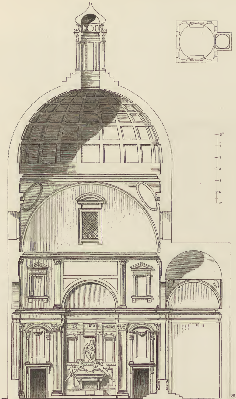
Fig. 147. Medicische Capelle bei S. Lorenzo.
