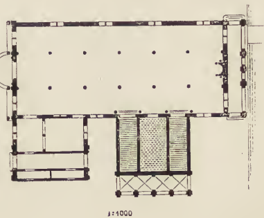
Fig. 157 und 158. Scuola di S. Rocco zu Venedig.
