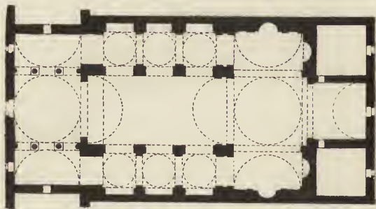
Fig. 188. Annunziata zu Arezzo. Grundriss. (Gnauth.)
