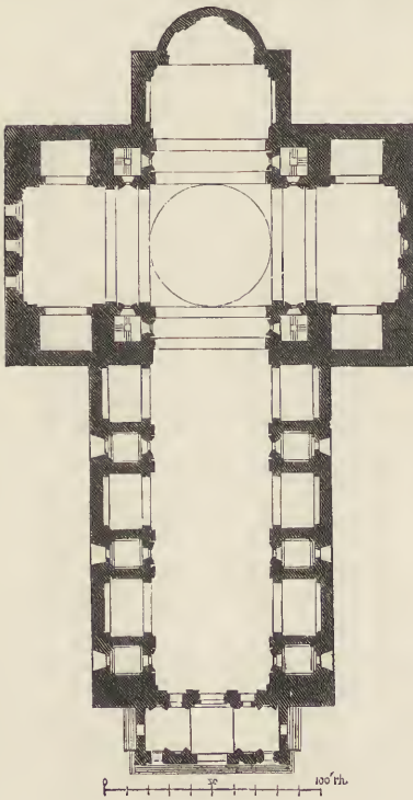
Fig. 119. S. Andrea zu Mantua.
