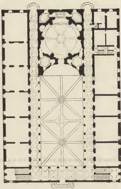
Fig. 153. Sapienza zu Rom. Grundriss. (Nach Gurlitt.)
