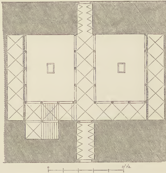
Fig. 167. Pal. Pizzardi zu Bologna. (L.)
