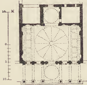
Fig. 67. Capp. Pazzi zu Florenz. Grundriss. (Nach Paulus.)
