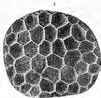
Michelinia furvosa de Kon. Kohlenkalk. Tournay. Belgien. A Stock von oben, B von unten, C Vertikalschnitt (nach Gaudry).
