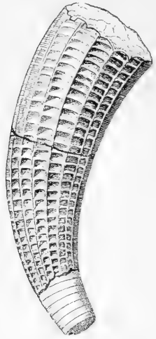
Fig. 1045. Cyrtoceras corbulatum Barr. Ober-Silur (E). Dvoretz, Böhmen. (Nach Barrande.)
