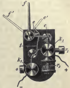
Fig. 375. Contactvorrichtung.
