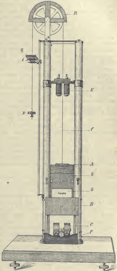
Fig. 342. Falltachistoskop.
