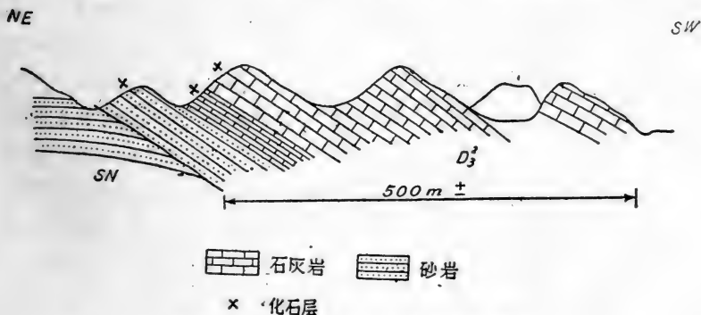
图8. 宜北治安乡东北三里泥盆纪地层
