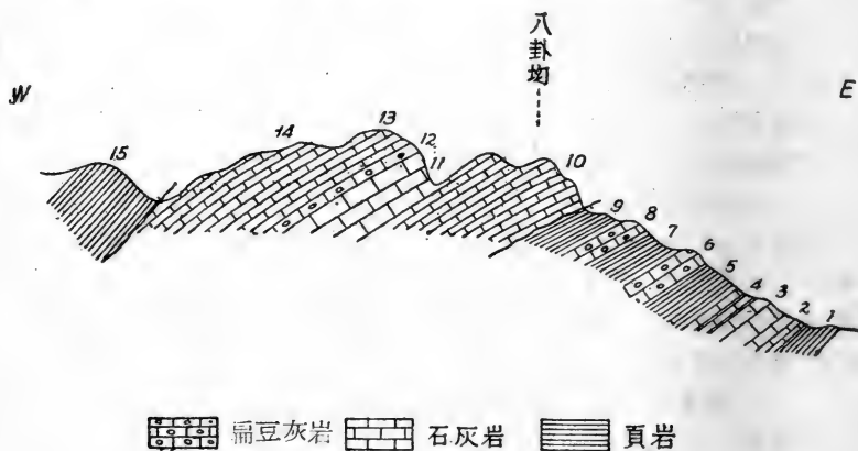
图 32. 河池西八卦坳剖面
