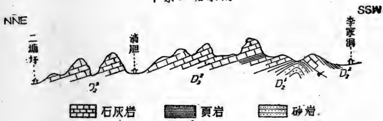
图 17. 平乐二塘东南地层剖面
