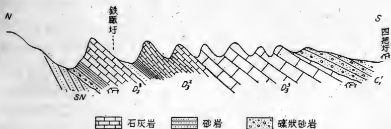
图7. 天河东二十里铁厂圩至罗城四把圩泥盆纪地层剖面
