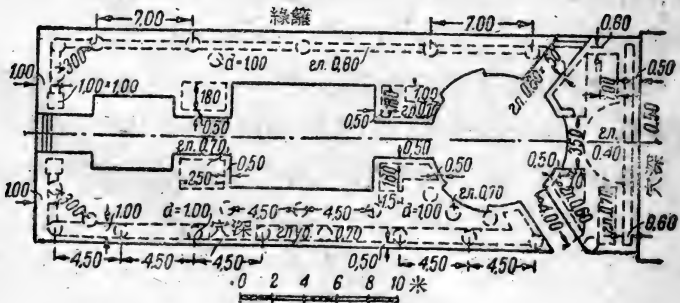
圖 157. 栽植施工圖(單位:米)。
