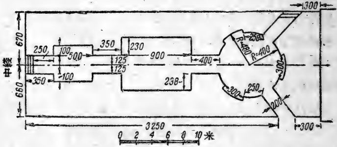
圖 156. 布置圖。
