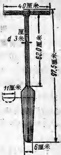
圖 120. 科列索夫植樹鉞。
