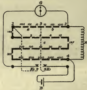
188. London P. O.
