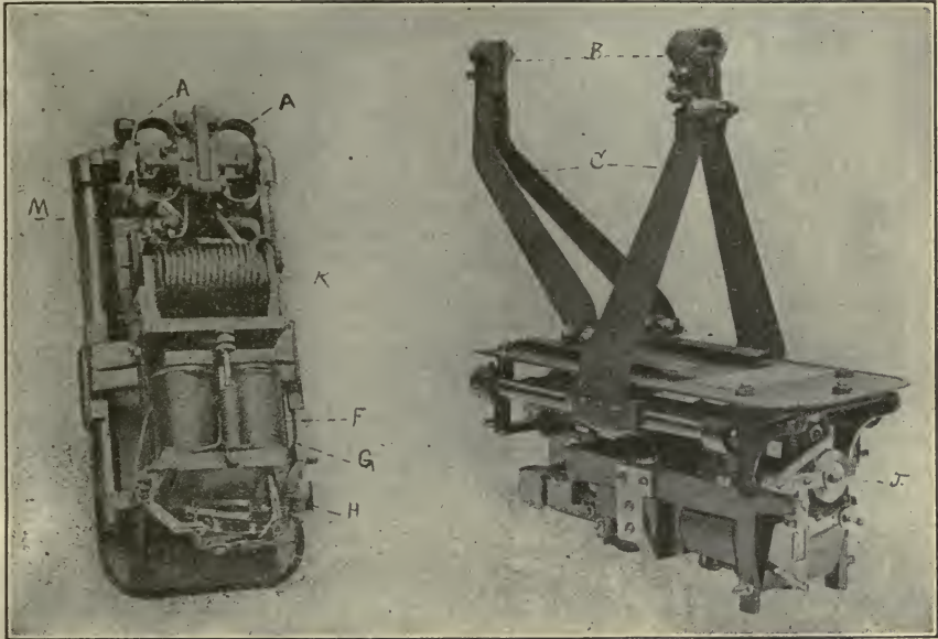
127. G. E. Search Light.
