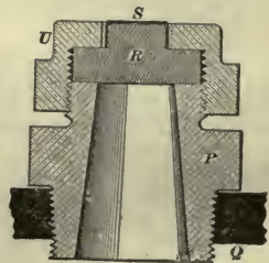
7. Fusible Plug.
