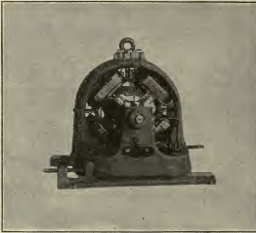
99. W-e Multipolar.
