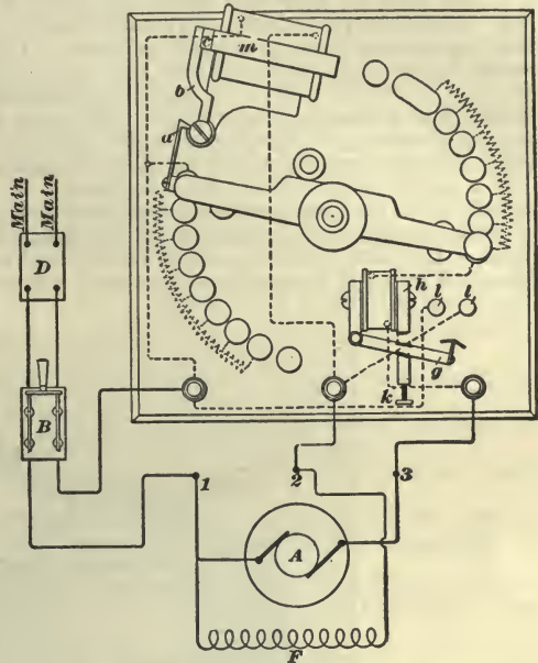
111. Automatic O. L. and U. L. Circuit Breaker.
