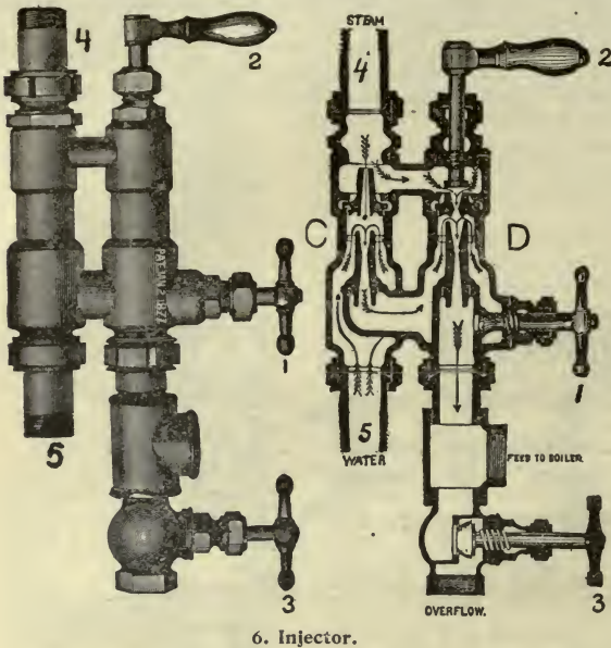
6. Injector.
