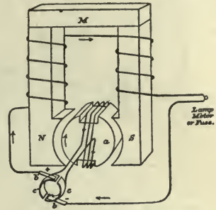
39. Simple D. C. Dynamo.
