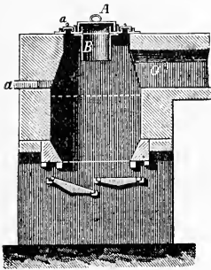
FIG. 141.—Gas generator.
