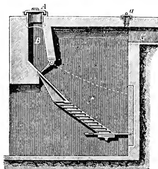
FIG. 143.—Gas generator.
