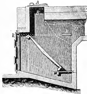
FIG. 142.—Gas generator.
