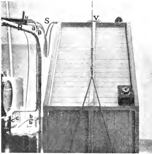
Ansicht der Grafeschen Respirationskammer in geschlossenem Zustande. (Buchstabenklärung im Text.)
