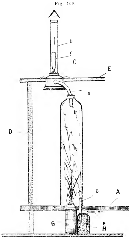
Hellriegels Apparat zur Bestimmung des Einflusses der Luftfeuchtigkeit auf den Ernteertrag nach Bürgerstein 1. c.
