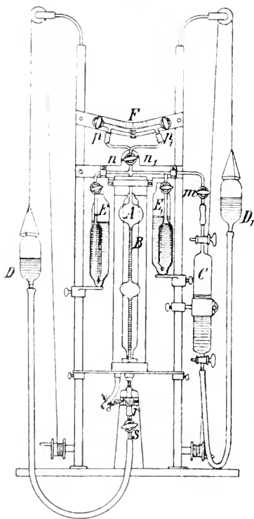
Gasanalyse-Apparat nach Peterson-Hogland-Tobiesen zur Analyse der nach dem Jaquet -schen Prinzipie entnommenen Teilluftströme. (Genauere Beschreibung der Apparatur und Methodik im Text.)
