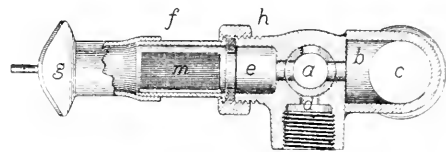
Durchschnitt durch Dreiwegventil. Anfeuchter und Mundstück auf \frac{2}{3} verkleinert. Das Dreiwegventil (a) ist durch ein T-Stück (b) mit dem Hauptluftrohre (c) verbunden. Das Mundstück (g) ist an dem den Anfeuchter (m) enthaltenden Metallrohre befestigt, das an das Dreiwegventil geschraubt wird.
