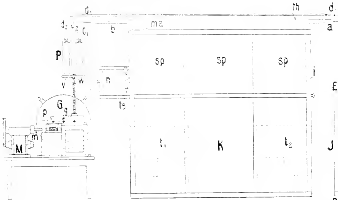
Gesamtansicht des Respiationsapparates von Stähelin und Kessler. (Kammer in Vorderansicht.)
