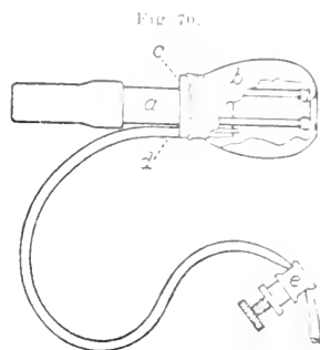
Benedictsche Nasenolive. Ein Gummifingerling (b) ist an einem Glasrohr (a) festgebunden und mit Luft aufgeblasen, die durch eine kleine, durch den Gummipropfen gesteckte Glasröhre gepreßt und mit einer Klemmschraube (e) festgehalten wird.
