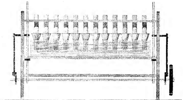
Dardscher Apparat zur Beobachtung schwacher Trübungen.
