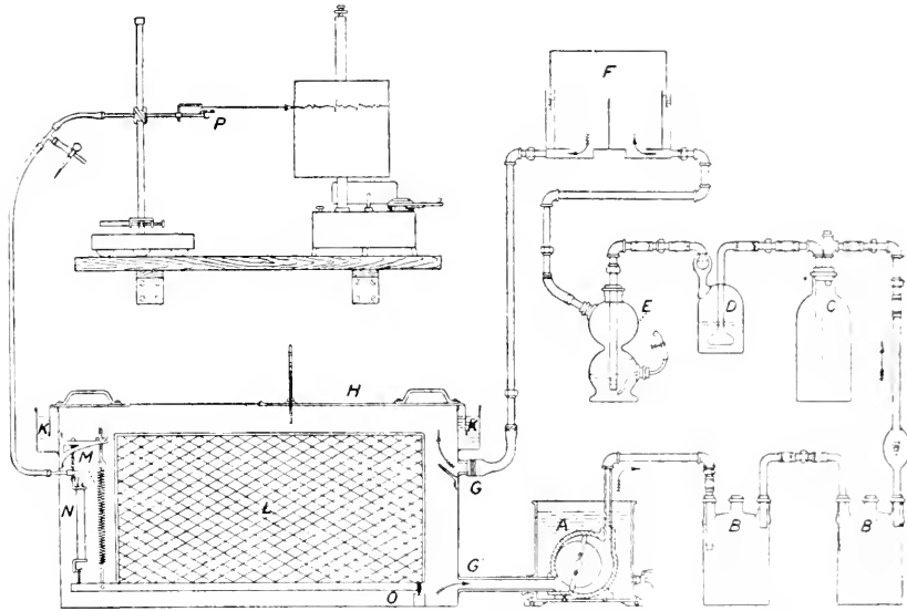
Ansicht der Benedict'schen Apparatur mit Einschaltung einer Kammer für Versuche mit Tieren oder Säuglingen. Rotationspumpe (A), Woulff'sche Flaschen (B und B'), Natronkalkflasche (C), Schwefelsäureflasche (D), Luftanfeuchter (E), Spirometer (F) und Verbindungen (G, G') mit der Respirationkammer. Der Käfig oder das Bott (L) ruht auf der einen Seite auf Schneiden (O) und die andere Seite wird von einer starken Feder (M) gehalten. Ein Pneumograph (N) stellt die Verbindung mit dem Tambour (P) her, der auf einem Zylinder schreibt. Der Kasten wird durch den Deckel (H) verschlossen, der in den Wasserverschluß (K, K') paßt.
