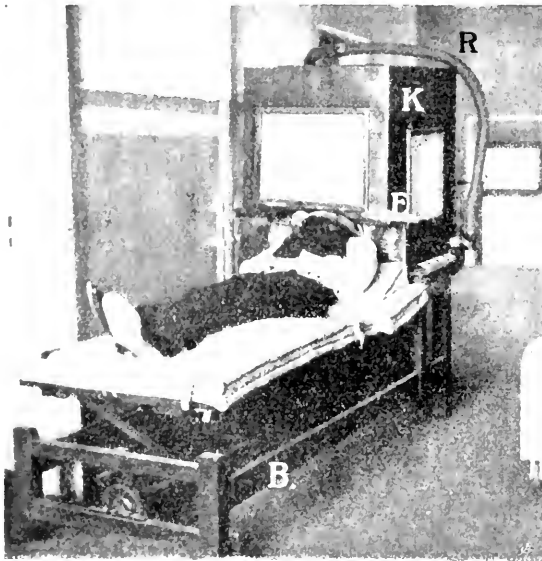
Gesamtansicht des Kopfrespirationsapparates von Grafe. B Versuchsbett, das aus drei Teilen besteht, die durch besondere Kurbelvorrichtungen in jede beliebige Lage zueinander gebracht werden können. K Kopfkasten mit Halsausschnitt, an dem die Gummihalskrawatte des Kranken befestigt wird, und Scheibe E Stelle für den Eintritt der Luft. R biegsames Metallrohr zur Verbindung mit der Gasuhr (nicht mit abgebildet).
