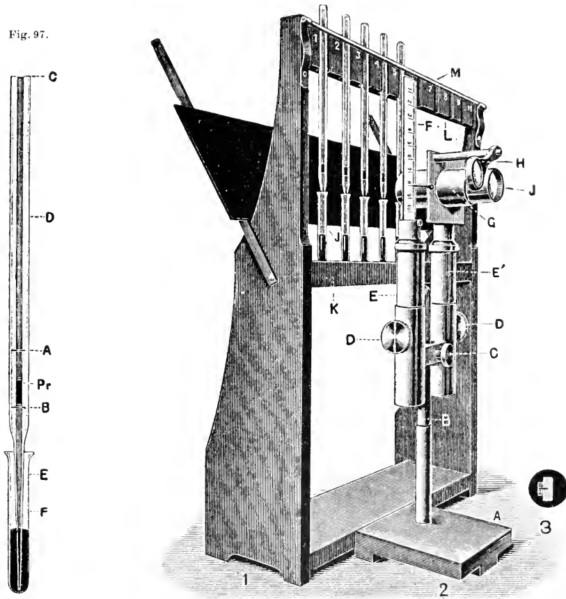
Apparat zur genauen quantitativen Bestimmung von Präzipitaten nach G. Nuttall und O. Inchley.
