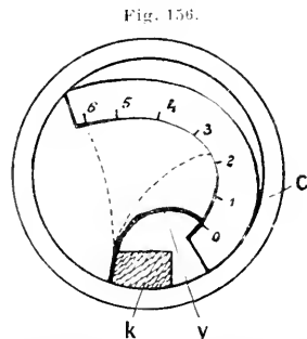
Fig. 156. F. Darwins Yucca-Hygroskop. Die gestrichelten Linien zeigen die sukzessive Aufrollung des Yucca-Streifens infolge Feuchtigkeit.
