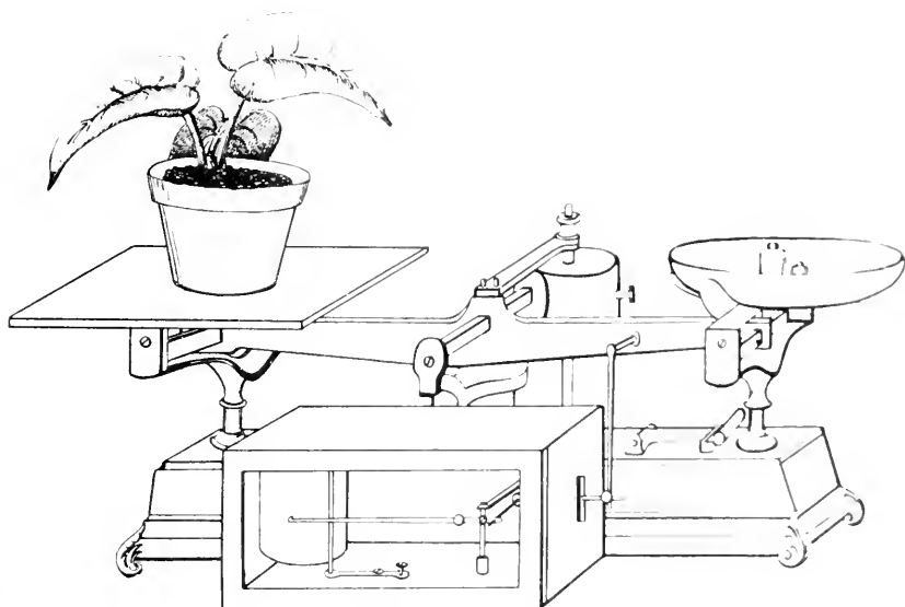
Evaporimetre enregistreur von Richard Feilke, Paris.
