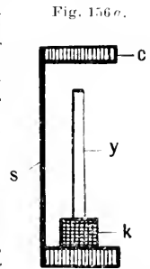
Fig. 156 c . F. Darwins Yucca-Hygroskop in der Aufsicht.
