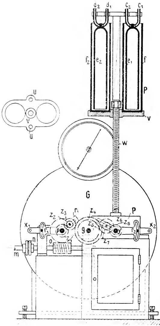
Die Vorrichtungen zur Entnahme der Teilströme an dem Respiationsapparate von Stahlbin und Kessner. (Erläuterungen im Text.)
