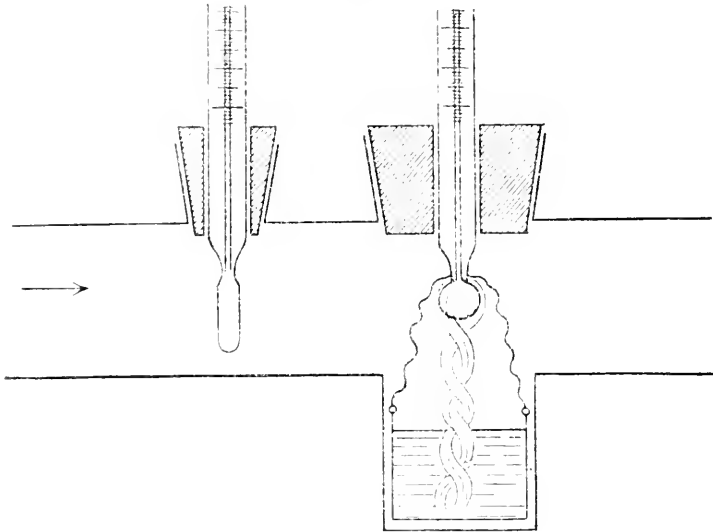
Die Anordnung der Psychrometer zur Bestimmung der Wasserdampftension in dem Apparate von Stübelin-Kossner .
