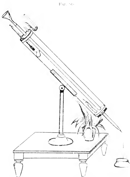
Alois Apparat zur Bestimmung des Einflusses der Lufttemperatur auf die Transpiration nach Aloi (Fig. 168).
