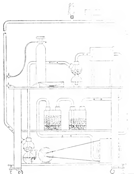
Schematische Abbildung der sämtlichen Anordnungen der einzelnen Teile des Benedictschen Apparates. (Die Pfeile geben die Ventilationsrichtung an.)
