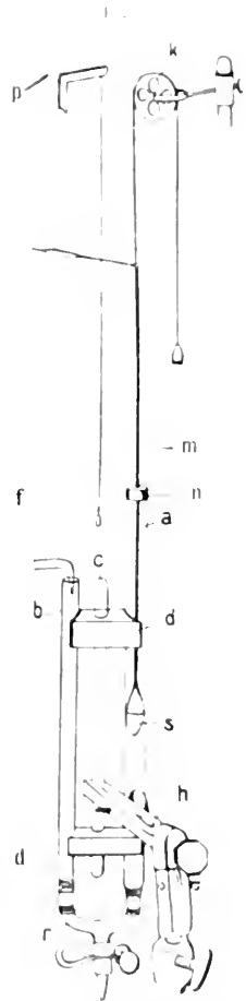
Fig. 1. Apparat zur Beobachtung der Gas- und Wasserbewegung in der Pflanze. (M. v. L. 1887.)
