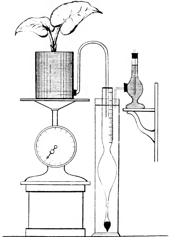
Apparat von Krutitzky, nach Burgerstein 1. c.
