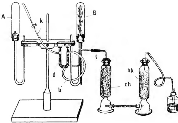
Verschaffells Apparat (Einfluß der Kohlensäure auf die Wasserdampfabgabe) nach Burgerstein l. c.
