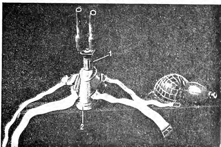
Gesichtsmaske von Rolly und Rosiewicz. 1 stellt das Verbindungsrohr nach dem Respirationsapparate dar, 2 einen aufblasbaren Gummischlauch, der im Versuche das Gesicht (Mund- und Nasengegend) luftdicht abschließen muß.
