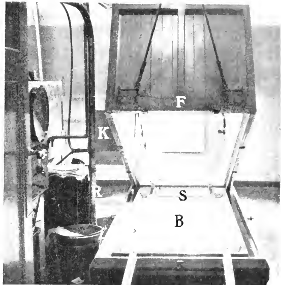
Ansicht der Grofesch Respirationskammer in geöffnetem Zustande.
