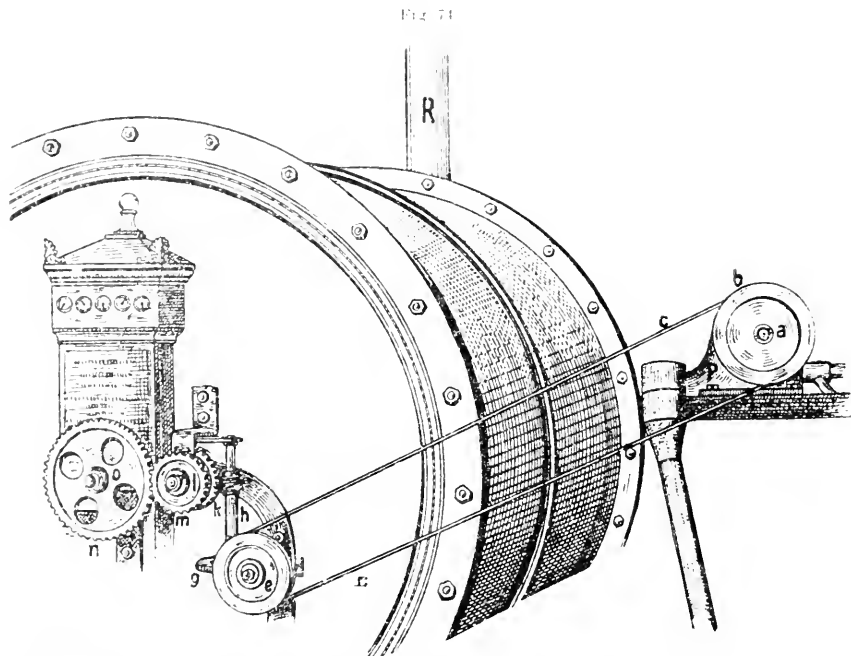
Fig. 73. ist über die Antriebsvorrichtungen für die Gasuhr und die Entnahme der Teilströme an dem Rubnerschen Apparate. (Buchstabenklärungen vgl. den Text.)
