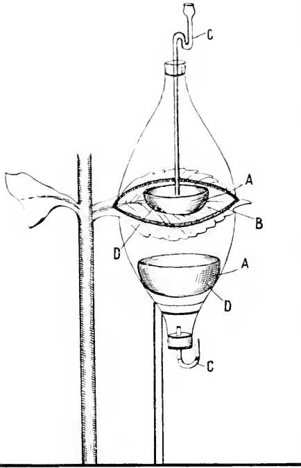
Garreus Apparat zur vergleichenden Bestimmung der Transpirationsgröße von Blattober- und -unterseite (nach Burgerstein l. c.).
