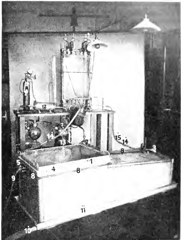
Ansicht der Respirationskammer von Rolly für langdauernde Versuche. Der Kasten in das auf S. 160 u. ff. beschriebene Respirationssystem eingeschaltet. Ein Patient (b) liegt im Kasten. (Weitere Zahlenerklärungen im Text.)
