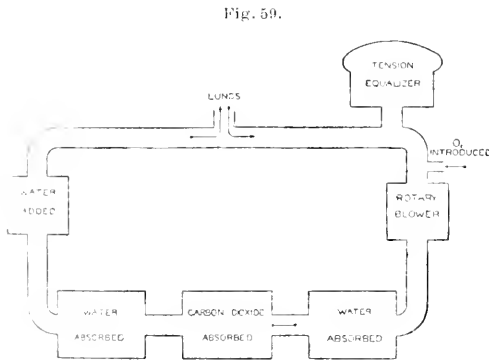
Schema der Anordnung des Benedict'schen Apparates.
