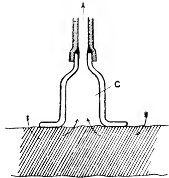
Die auf das Blatt aufgeklebte Glaskammer c vergrößert. Porometer von Darwin und Pertz .
