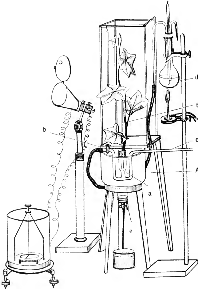
Vesques Apparat zur Messung der Absorption.
