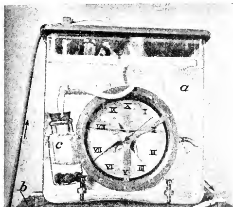
Bohrsche , unter Wasser stehende Gasuhr. Der in die Röhre kommende Sauerstoff geht zuerst in die kleine Flasche ( c ) und dann in die in dem Glasgefäße ( a ) unter Wasser stehende Gasuhr. Das Brett ( b ) dient zum Nivellieren der Gasuhr.
