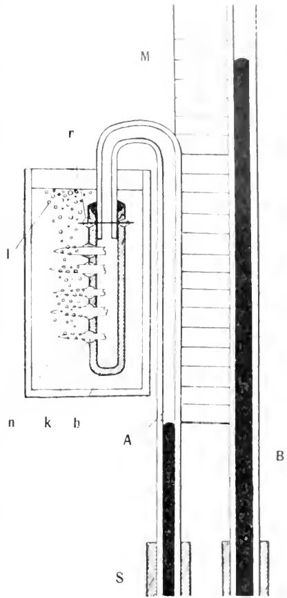
1. Dengler's Apparat zum Einführen von Wasser in die Spaltöffnungen. a. Bleirohr, b. Drehungsstellen der Nadeln, c. Nadeln, A. fester Manometer (blechbeschreibbarer Manometerschlauch), B. Druckschlauch, der beide verbindet, C. Druckschlauch, der beide verbindet, D. Verbindung zwischen Bleirohr und Nadeln, beide durchbohrend, E. Unterwasserbehälter, in dem die Nadeln austretend abgelesen werden.
