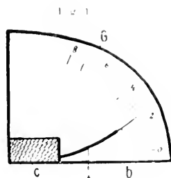
E. Darwins Horn-Hygroskop.
