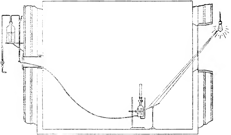
Vorrichtungen zur Verbrennung von Alkohol bei der Prüfung der Leistungsfähigkeit großer Respirationsapparate. (Anordnung nach Atwater und Benedict .)
