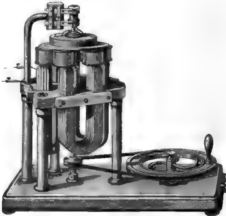
Fig. 36. Störers verbesserte Maschine.
