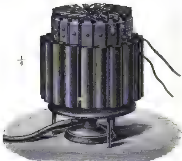
Fig. 30. Noë's Thermosäule.
