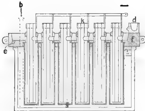
Fig. 168. Zelle zur Elektrolyse von Bromiden nach Wünsche.
