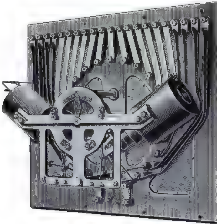
Fig. 143. Grosser Doppelselbstzellschalter der Akkumulatorenfabrik Hagen & W. Hinteransicht.
