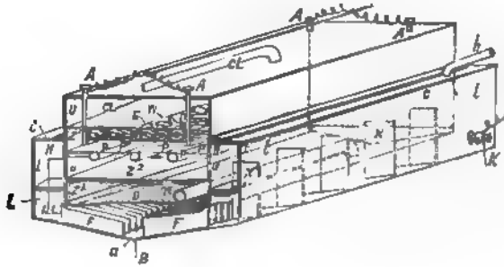
Fig 217. Elektrolyseapparat von Carmichael.
