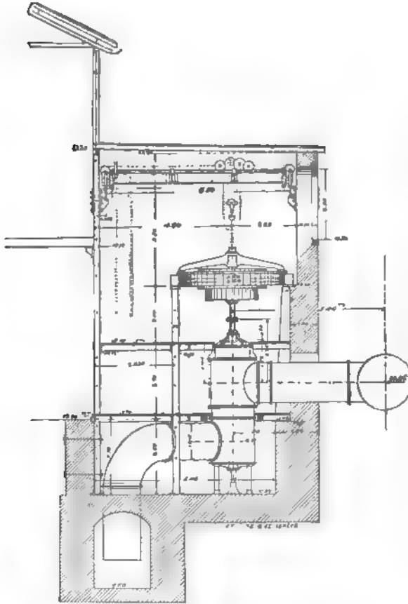
Fig. 277. Turbinenanlage der Aluminiumindustrie-Aktiengesellschaft in Neuhausen (Aufriß).
