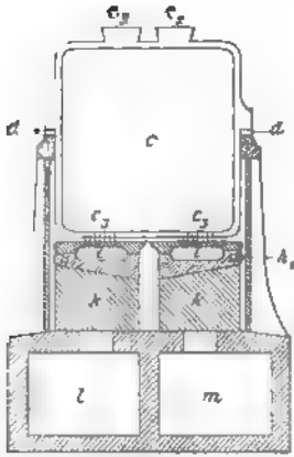
Fig. 281 Elektrolyseur Ferranti-Noad zur Bleiweißdarstellung
