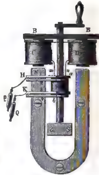
Fig. 35. Störhrs Maschine.
