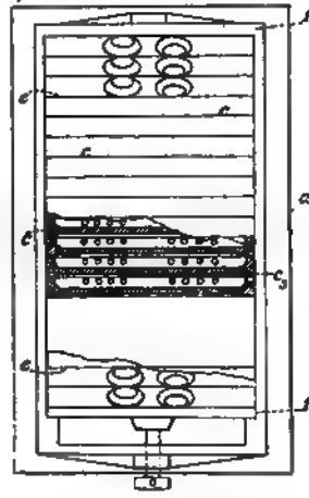
Fig. 281 Elektrolyseur Ferranti-Noad zur Bleiweißdarstellung
