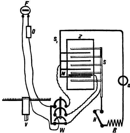
Fig. 71. Versuchsanordnung zur Messung der elektrischen Größen des Bleisammlers.
