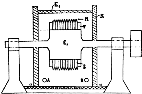
Fig. 201. Längsschnitt. Ottos Ozonisator (D.R.P. Nr 120688).
