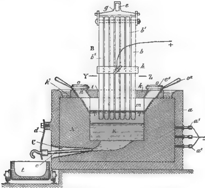
Fig. 178. Aluminiumgewinnung nach Héroult.
