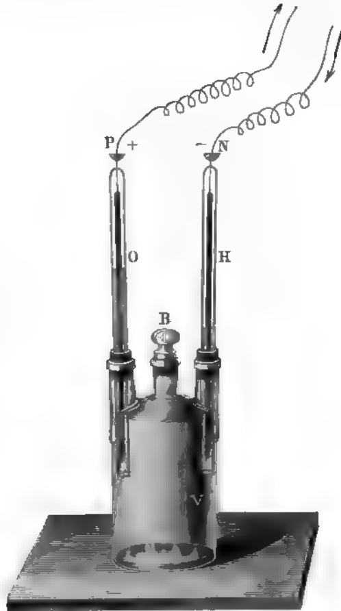
Fig 54. Groves Gasbatterie.
