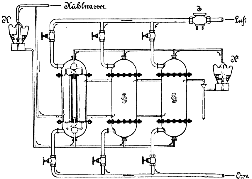
Fig. 205. Röhrenozonisator (Siemens & Halske).
