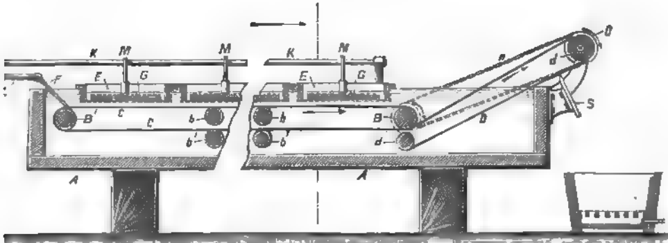
Fig. 273. Apparat von Möbius zur Scheidung von Silber und Gold.
