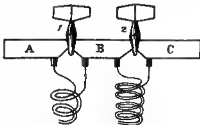
Fig. 123. Stöpselrheostat.
