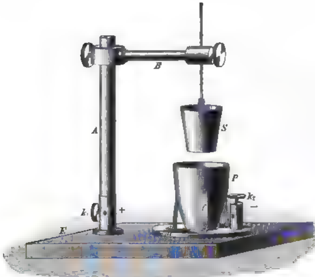
Fig. 94. Silbervoltameter.
