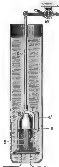
Fig. 97. Waterhouse- Elektrizitätsmesser.
