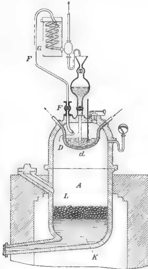
Fig. 230 Hulins Apparat zur Zerlegung von Alkalilegerungen mittels Wasserdampf.
