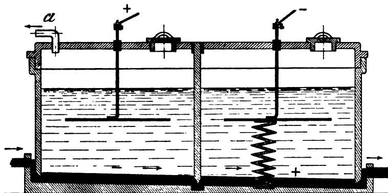
Fig. 249. Alkalichloridelektrolyse nach dem Quecksilberverfahren. (Bildungs- und Zersetzungszelle.)
