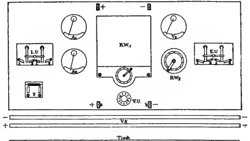
Fig. 167. Ansicht der Schaltanlage.
