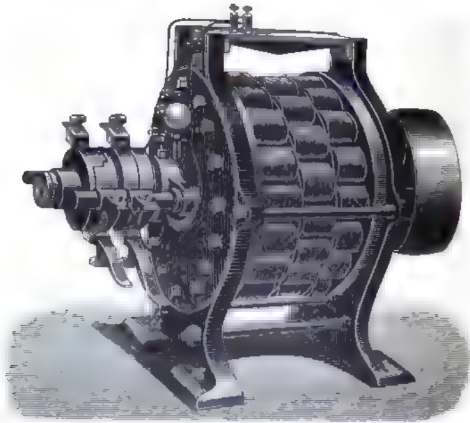
Fig 88. Maschine von Wilde
