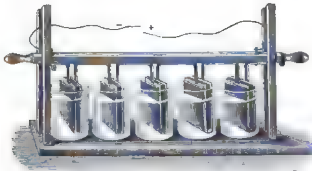
Fig. 5. Wollastons Batterie.
