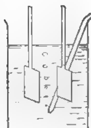
Fig. 98 Kupfervoltameter von Ostwald.
