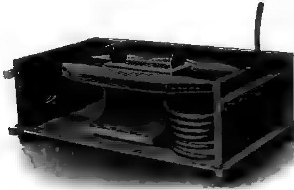
Fig. 257. Apparat zur Bereitung elektrolytischer Bleichlösung nach Haas-Oettel.
