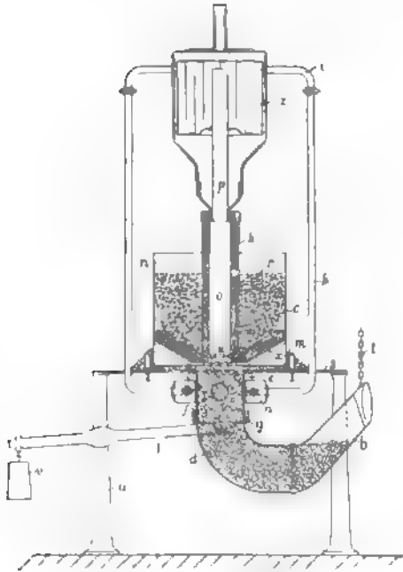
Fig. 216 Siemens' Karbidofen.
