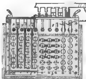
Fig. 235. Apparat zur Zerlegung von Chloralkalien der Soc. Outhenin Chalandre Fils & Cie.
