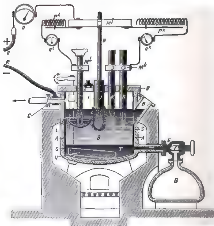
Fig. 229. Hulin's Apparat zur Herstellung von Alkalilegerungen mit Schwermetallen
