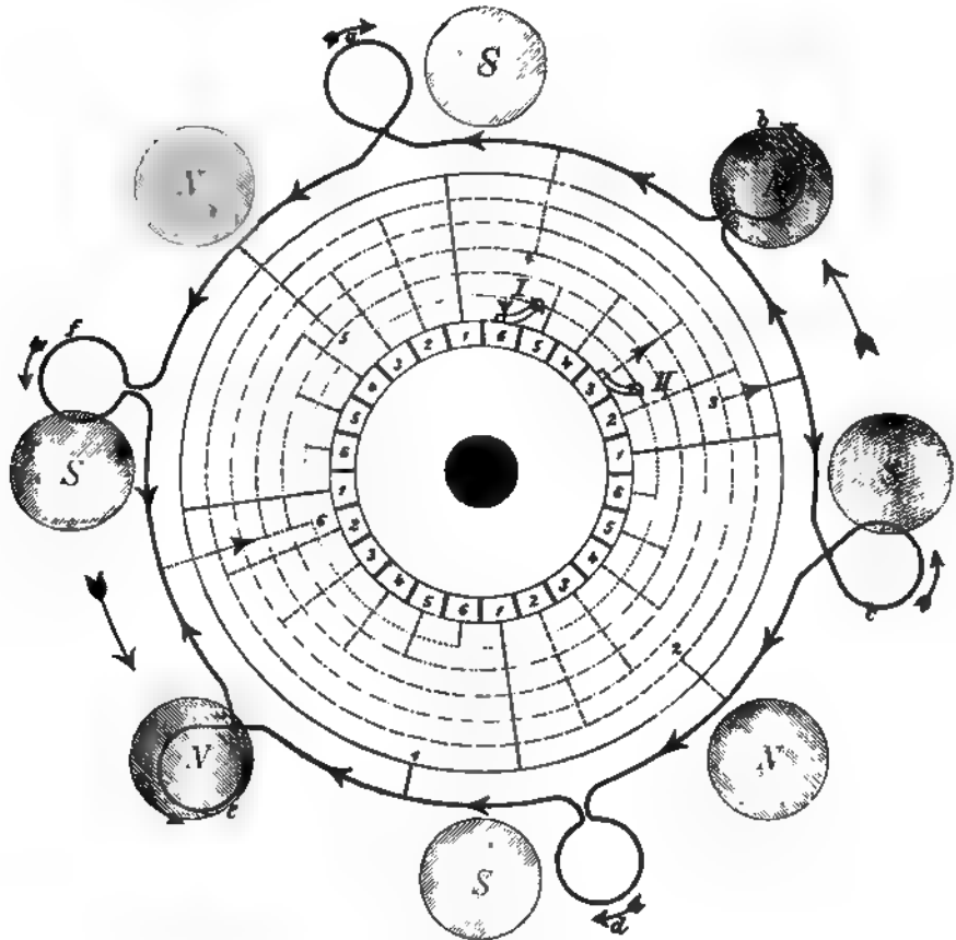
Fig. 44. Gleichstrommaschine von Hefner-Alteneck. Verbindung der Armaturespulen unter sich und mit dem Kommutator.
