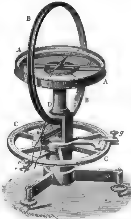
Fig. 79. Sinussbussole.
