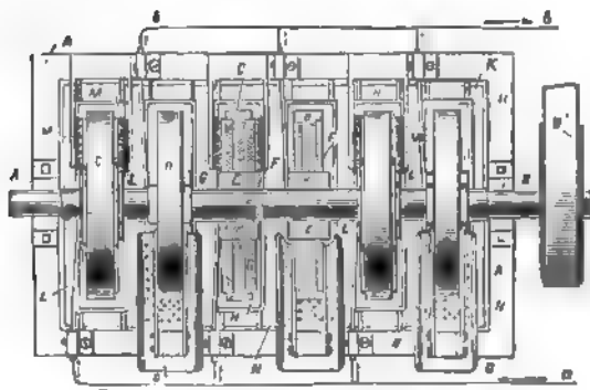
Fig 289 Apparat zur Silberaffination: Grundriss.
