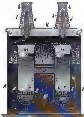
Fig. 24. Normalelement von Weston.
