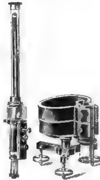
Fig 86. Spiegelgalvanometer nach Deprez-d'Arsonval von Gaus und Goldschmidt-Berlin.
