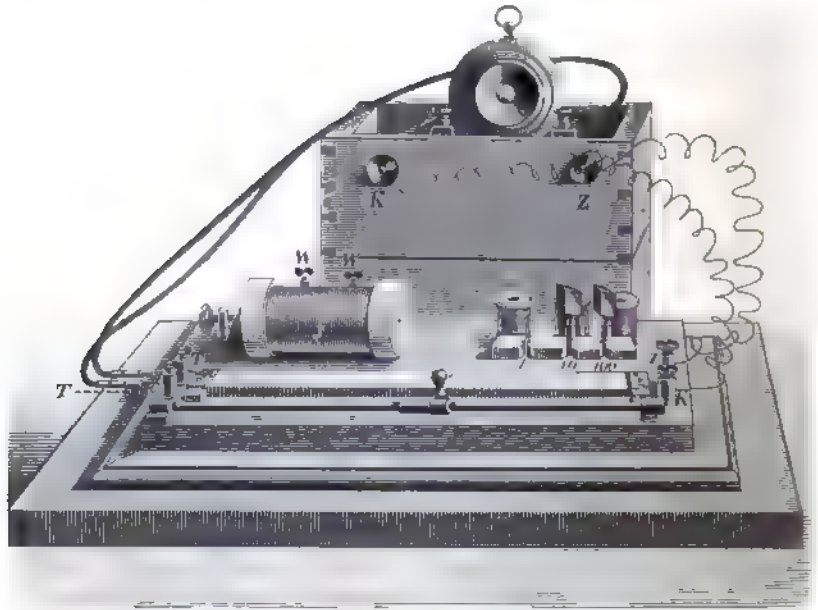
Fig. 113. Meßbrücke nach Kohlrausch.
