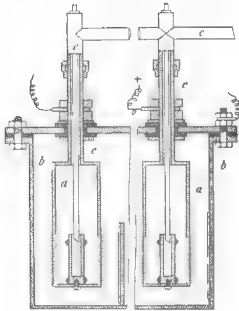
Fig. 191. Apparat zur elektrolytischen Darstellung von Fluor.
