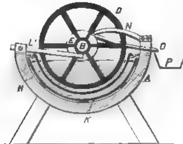
Fig. 268. Apparat zur Silberraffination: Vertikalschnitt
