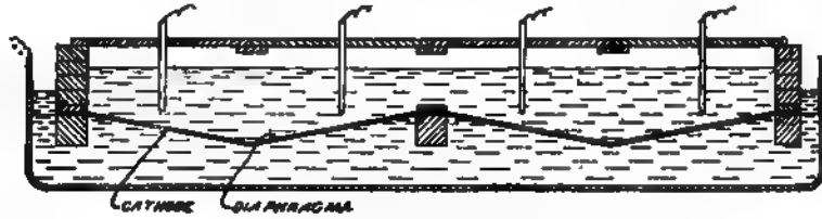
Fig. 245. Le Sueur-Zelle.
