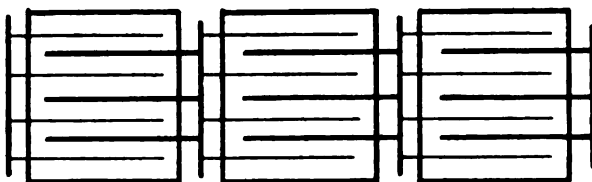
Fig. 64. Schaltung bei grossen Elementen.
