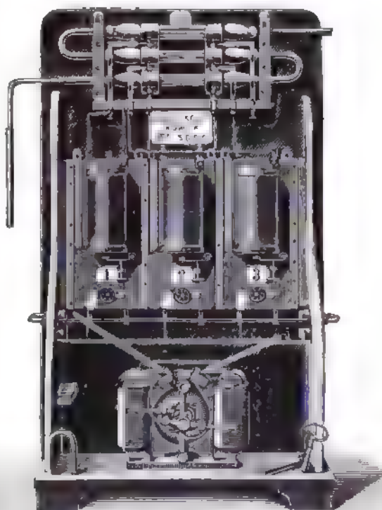
Fig. 195. Ozonisierapparat von Séguy.
