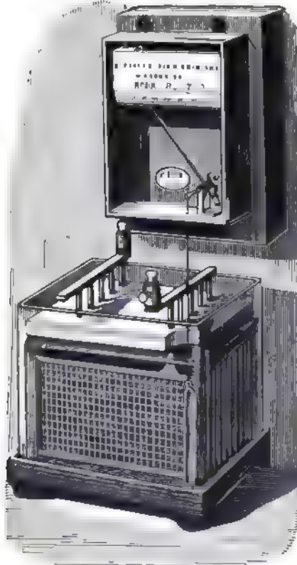
Fig. 73. Ladungs- und Entladungsanzeiger für Akkumulatoren.
