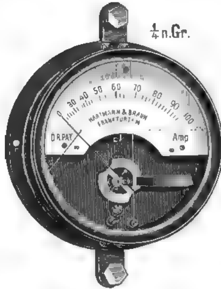
Fig. 92. Hitzdrahtampèremeter.
