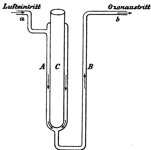
Fig. 194. Ozonisorator.
