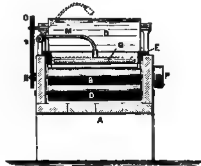
Fig. 275. Apparat von Möbius zur Scheidung von Silber und Gold.
