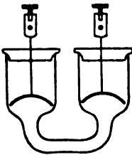
Fig. 114. Widerstandsgefäße für gutleitende Flüssigkeiten.
