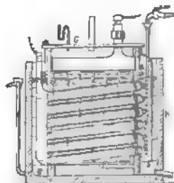
Fig. 235. Apparat zur Zerlegung von Chloralkalien der Soc. Outhenin Chalandre Fils & Cie.
