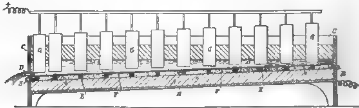
Fig. 222. Karbidofen der Gesellschaft „Volta“.
