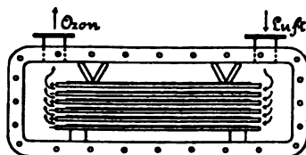
Fig. 304. Plattenozonisorator (Siemens & Halske).
