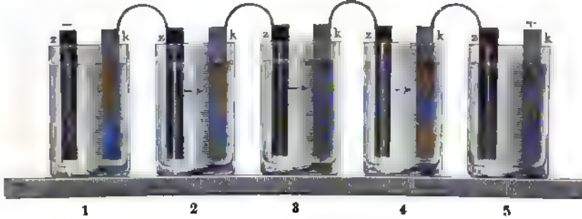
Fig. 2. Voltas Becherapparat.
