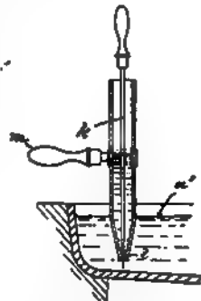
Fig. 237. Ausschöpfvorrichtung zum Apparat der Aluminiumindustrie A.-G. Neuhausen.
