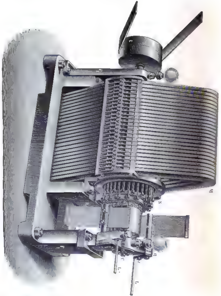
Fig. 49. Trommelmaschine von Hefner-Alteneck.
