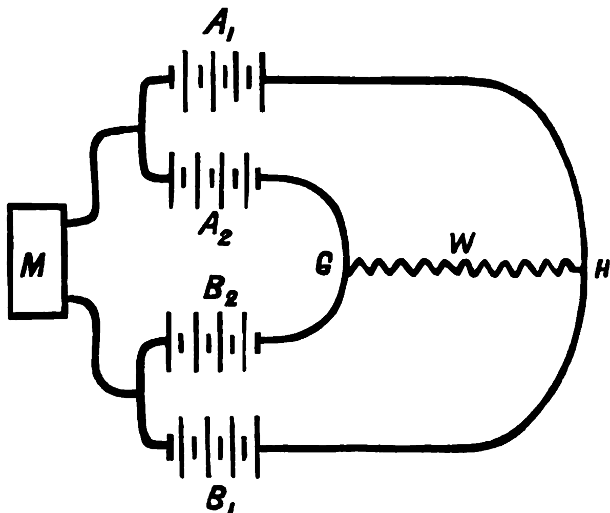
Fig. 53. Umwandlung von Wechselstrom in Gleichstrom nach Grätz.
