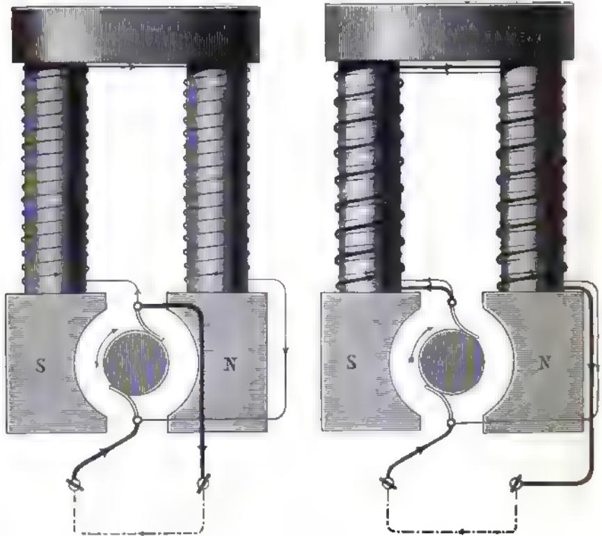
Fig. 47. Schaltung der Nebenschlussmaschine.
