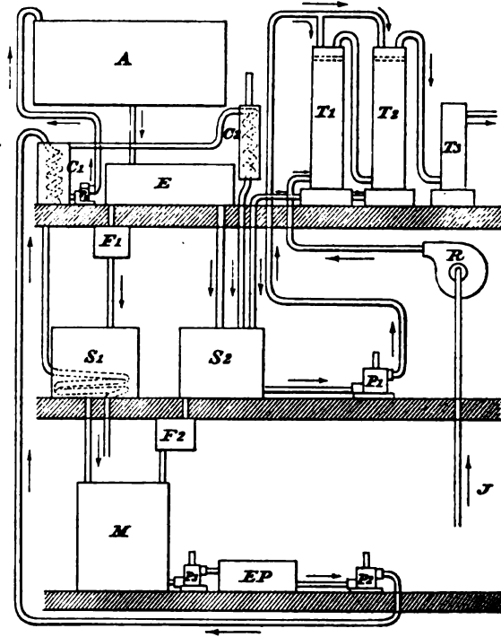
Fig. 280. Bleiweißgewinnung nach Ferranti-Noad.
