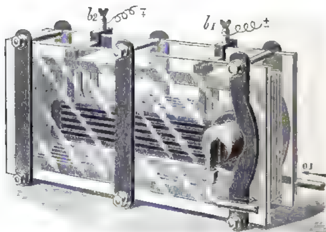
Fig 136 Ozonisator von Otto.
