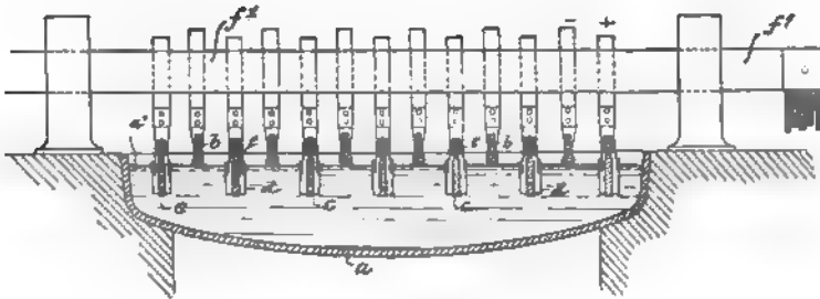
Fig. 236. Natriumgewinnung der Aluminiumindustrie A.-G. Neuhausen.
