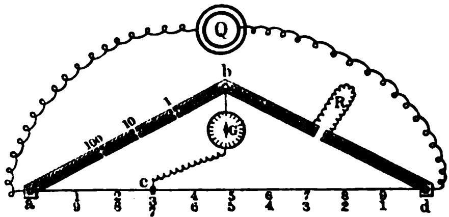
Fig. 112. Kirchhoffsche Brücke.
