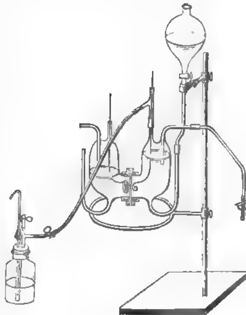
Fig. 291. Elektrolyseapparat nach Hofer.
