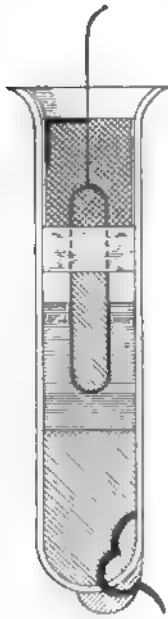
Fig. 21. Normal-element nach Rayleigh.
