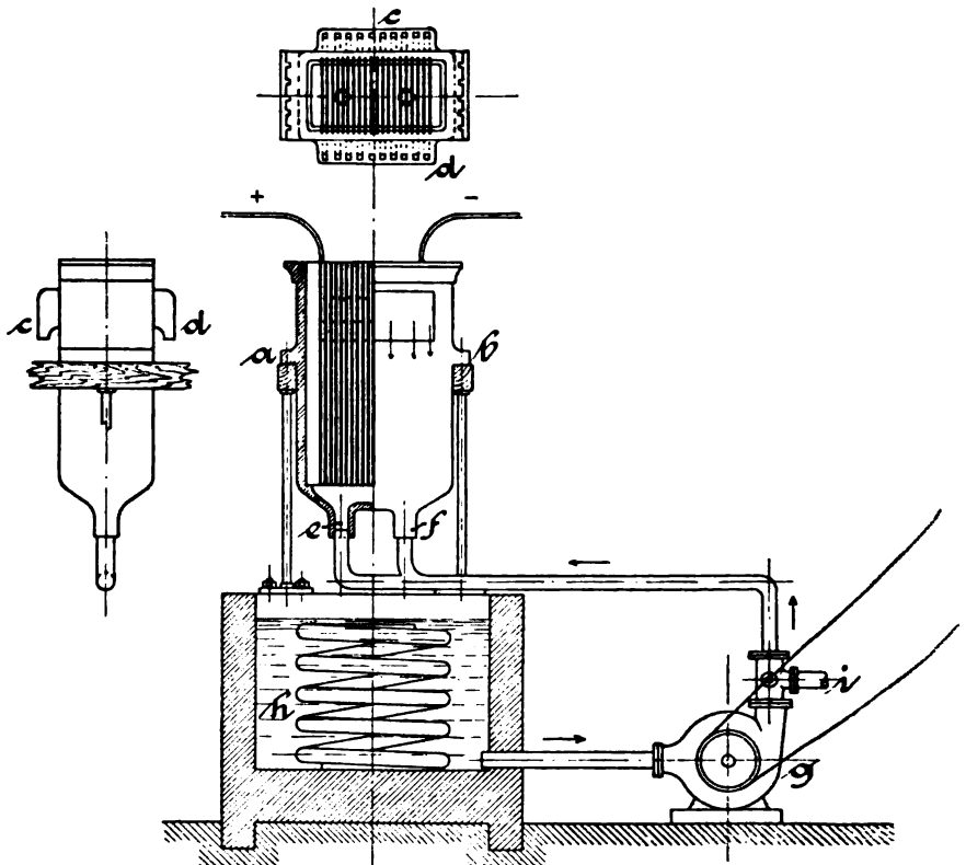
Fig. 256. Apparat zur Gewinnung elektrolytischer Bleichlösung nach Kellner.
