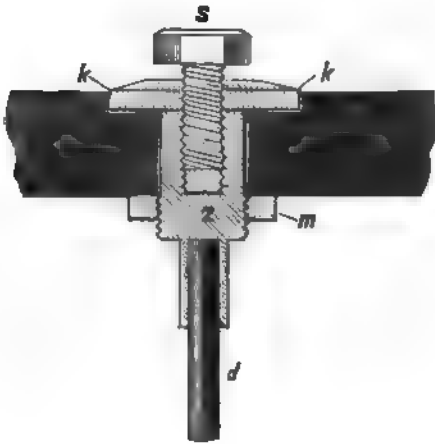
Fig. 148. Polkontakt.
