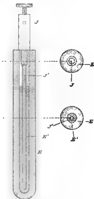
Fig. 279. Anode zum Elektrolyseur Lyte.
