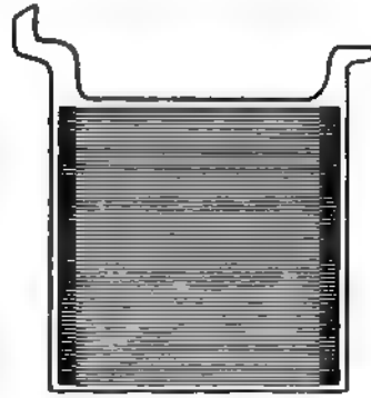
Fig. 58. Positive Tudor-Platte.
