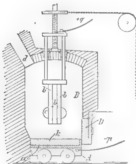
Fig 211. Tenners Karbidofen
