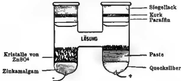
Fig. 22. Normalelement von Clark. (M-Form nach Lord Rayleigh)
