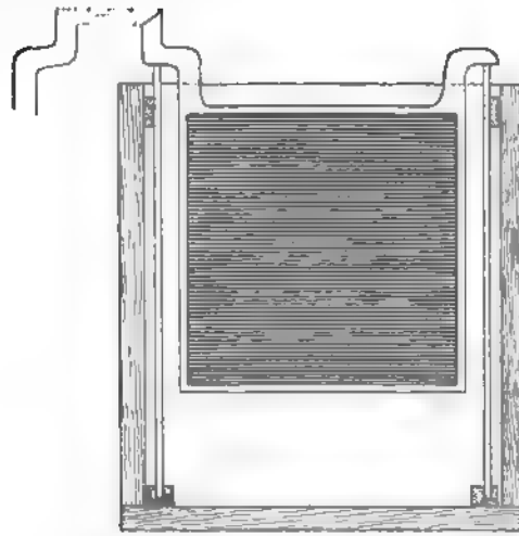
Fig. 68. Elektrode für grössere Zellen
