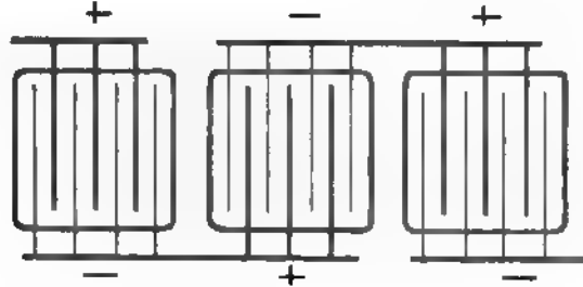
Fig. 69. Schaltung bei kleineren Zellen.
