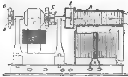
Fig 197 Ozonisierapparat von Tesla.
