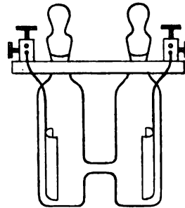
Fig. 114. Widerstandsgefäße für gutleitende Flüssigkeiten.
