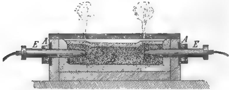
Fig 171. Cowies-Ofen zur Darstellung von Aluminiumlegierungen.
