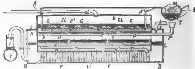
Fig. 246. Elektrolyseapparat von Carmichael.
