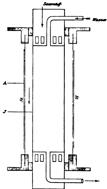
Fig. 193. Ozonapparat von Siemens.
