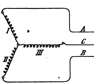
Fig. 49. Offene oder Sternschaltung.
