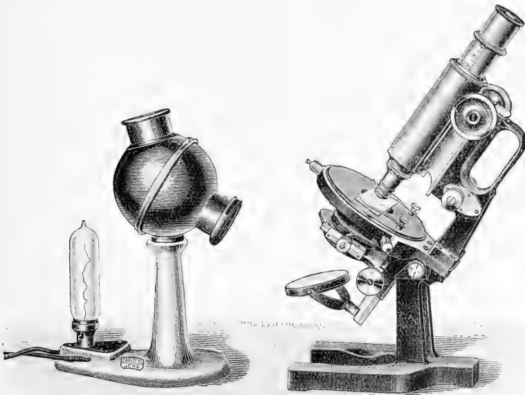
Fig. 3. Paraboloidkondensator (eingeschaltet) mit Nernstlampe (Zeiß-Jena).
