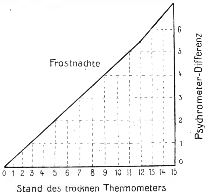
Fig. 186. Nachtfrostkurve nach LANG.
