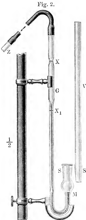
Viskosimeter (nach Hirsch u. Beck). Z Saug- und Druckrohr, durch welches das in M gebrachte Blut in G hinaufgesogen und aus G wieder herausgedrückt wird. Die Zeit, welche nötig ist, damit der Meniskus von X bis X 1 fällt, wird gemessen. V Verschlussrohr mit Schloß SS , um das Ganze sofort nach Einbringen d's Blutes in das Thermostatwasser einsetzen zu können.
