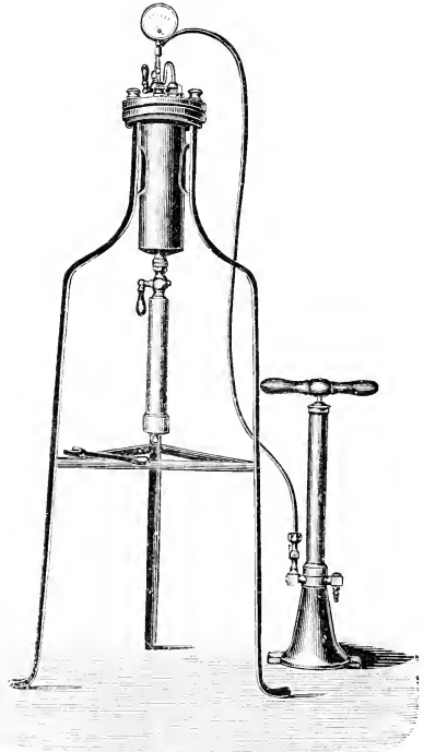
Fig. 76. Chamberland-Filter, mit Druckluftpumpe rechts montiert. — Ca. ein Zehntel der nat. Größe.
