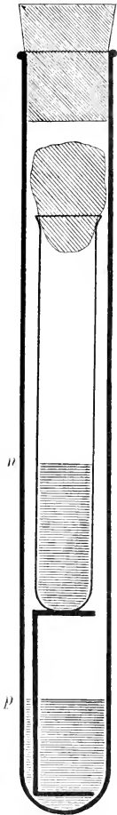
Fig. 88. BUCHNER'S Anaerob-Röhre. Bei p die Pyrogallol-Lösung, darin das Drahtbänkchen, auf diesem das Reagensglas mit dem beimpften Nährboden ( n ). Etwas verkleinert. Nach BUCHNER.
