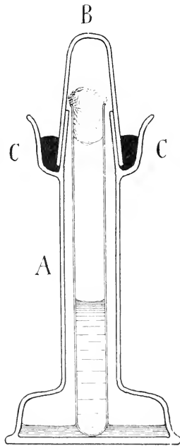
Fig. 89. OMELJANSKI'S Vorrichtung zur Züchtung Anaerob. Erklärung im Text.
