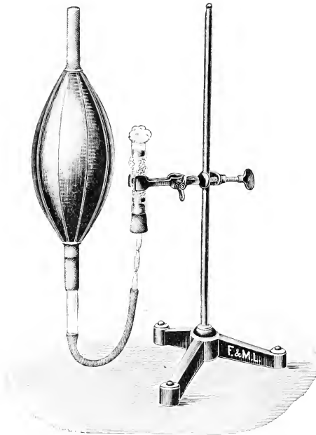
Fig. 75. Luftuntersuchungs-Apparat nach FICKER, bestehend aus der Ballonpumpe (links) und dem mit Glassand beschickten Filterröhrchen (rechts).
