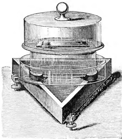
Fig. 78. Plattengießapparat, bestehend aus Nivelliergestell, weiterer und engerer Glasschale, Glasscheibe zur Aufnahme der Platten und Glasglocke zum Bedecken der letzteren. — Ungefähr ein Fünftel der nat. Größe.
