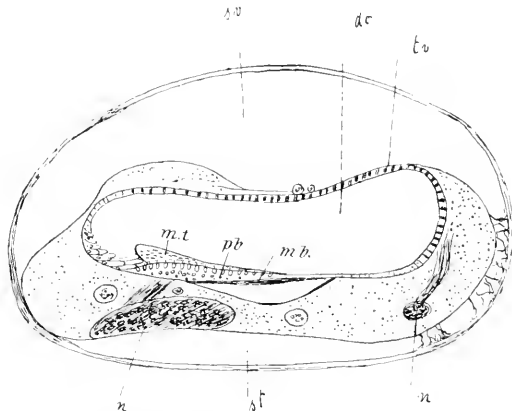
Fig. 123. Schnitt durch den Ductus cochlearis der Taube (nach RERZIUS 1881). d.c. Ductus cochlearis. p.b. Papilla basilaris. m.t. Membrana tectoria. v. Nerv. s.v. Scala vestibuli. s.t. Scala tympani.
