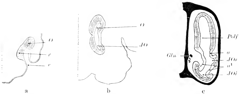
Fig. 50a—c. Schnitte durch das Riechorgan von Chrysemys picta von 5 mm Länge (a, Vergr. 40:1), 5 mm Schildanlage (b, Vergr. 30:1) und Emyd lut. von 14 mm Schildlänge (c). Nach SEYDEL (1896). a seitliche, a' mediale Grenzfalte, e Einführungsgang. Gln Glandula nasalis. JO JAKOBSON'sches Organ (SEYDEL) mit oberer ( JOs ) und unterer ( JOi ) Portion, angelegt als Rinne ( r ). O Hauptnasenhöhle. Polf Pars olfactoria.
