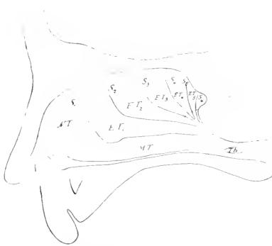
Fig. 72. Schema der Hauptmuschel und -furchen des menschlichen Foetus. Nach KILLIAN (1896). ET 1 — ET 5 1. bis 5. Ethmoturbinale. MT Maxilloturbinale. NT Nasoturbinale. S 1 — S 6 Hauptfurchen. Tb pharyngeale Tubenmündung.
