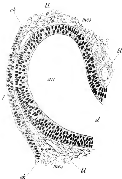
Fig. 208. Querschnitt durch die Augenanlage eines ungefähr 10-tägigen Kaninchenembryo. Nach RABL. Vergr. 200:1. au Augenblase. bl Blutgefäße. ek Ektoderm. l Linsenplatte. mes Mesoderm. st Stiel der Augenblase.
