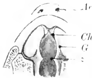
Fig. 63. Gaumen eines 3,8 cm langen menschlichen Foetus. Nach DURSUY (1869). Ac Apert. externa. Ch primitive Choanen, von den Gaumenfortsätzen ( G ) überwölbt, welche in ihrer Mitte zackenartig vorspringen (z), zur Anlage der Uvula.
