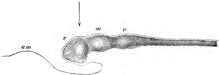
Fig. 163. Linkssseitige Profilansicht des Gehirns von einem Hühnerembryo aus der Mitte des 2. Brüttagcs, Vergr. 36:1. am Andeutung der Kopffalte des Amnion. m Mittelhirn. r Rautenhirn. v Vorderhirn. Der Pfeil bezeichnet die Lage des in Fig. 162 abgebildeten Schnittes.
