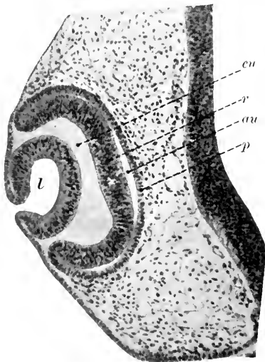
Fig. 192. Querschnitt der Augenanlage eines Hühnerembryo aus der Mitte des 3. Brütages. Präp. von M. HEIDENHAIN. Vergr. 100:1. l Lumen des Linsensäckchens. cu Augenbecherhöhle. r Retinalblatt. au Schventrikel. p Pigmentblatt.
