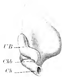
Fig. 38. Modell des rechten Geruchsackes einer Ichthyophislarve, ventral gesehen. Vergrößer. 25 : 1. Nach SARASIN (1890). Ch Choane. Chb Choanenschleimbeutel. UB unterer Blindsack.
