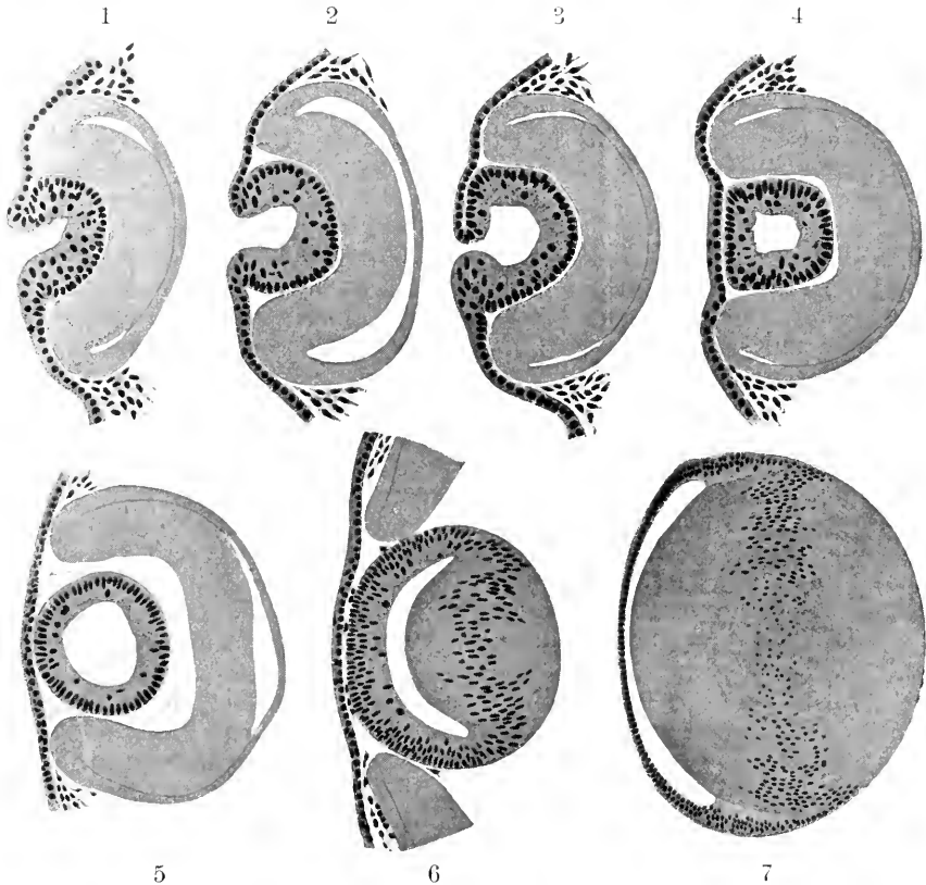
Fig. 189. Linsenentwicklung von Lacerta agilis . Nach RABL. No. 1—6 Vergr. 145:1, No. 7 Vergr. 90:1. Entwicklungsgrad der Embryonen: No. 1 24 Urvirbel; No. 2 27 Urvirbel; No. 3 28 Urvirbel; No. 4 29 Urvirbel; No. 5 33 Urvirbel; No. 6 48 Urvirbel, Körperlänge (im Bogen gemessen) 7—8 mm; No. 7 Körperlänge (im Bogen) 22 mm.
