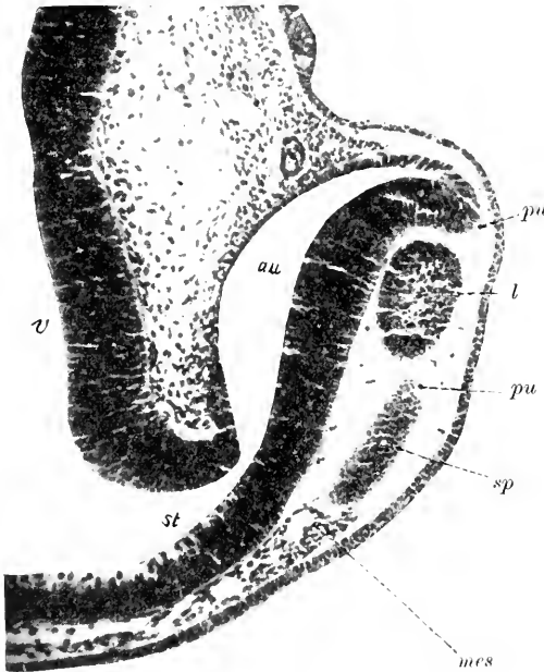
Fig. 233. Frontalschnitt durch das Auge eines Embryo von Torpedo marmorata von 14,5 mm Lange, 71 Urvirbel. Prap. von A. FRORIEP. Vergr. 100:1. au Sehventrikel. l Linse. mes Mesodermgewebe mit dem Augenbechergefa im proximalen Teil der Becherspalte. pu Pupillarrand des Augenbechers. sp rostrale Lippe der Augenbecherspalte, durch den Schnitt gestreift. st Ventrikel im Augenblasenstiel. v Ventrikel des Zwischenhirns.
