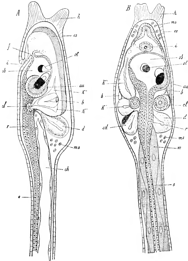
Fig. 152. Vorderer Körperabschnitt der frei schwimmenden Larve von Ascidia mammillata . Nach A. KOWALEWSKY (1871), aus KORSCHOLT und HEIDER's Lehrbuch. A Seitenansicht, B Dorsalansicht. au Auge (Sehepithel, Pigmentmasse und Linse mit Meniskus). ch Chorda. d Darmkanal. es Endostyl. f Flimmergrube. k , k' Kiementaschen. m Schwanzmuskeln. ms Mesenchymzellen. ot Otolith. r , s Medullarrohr. sb Sinnesblase (Gehirnventrikel?).
