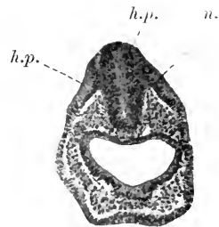
Fig. 77. Schnitt durch die Kopfgegend eines Embryos von Tropidonotus natrix . h.p. Hörplatte. n. Nervenrohr.
