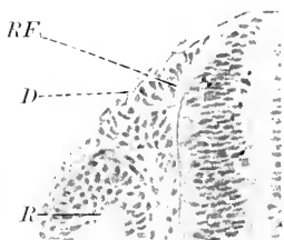
Fig. 15. Querschnitt durch das Riechfeld eines Forellen-Embryos, Stadium XI (KOPSCHE 1898). Vergr. 200:1. D Deckschicht. RF Riechfeld. R Retina.
