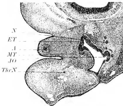
Fig. 70. Schnitt durch die Mitte des Geruchsorgans eines menschlichen Embryos von 15 mm Länge (Fig. 62). Vergr. 22,5: 1. A Auge. ET Ethmoturbinale I. JO JAKOBSON'SCHES Organ. MT Maxilloturbinale. N Nervus olfactor. Thr.N Thränenmasengang.
