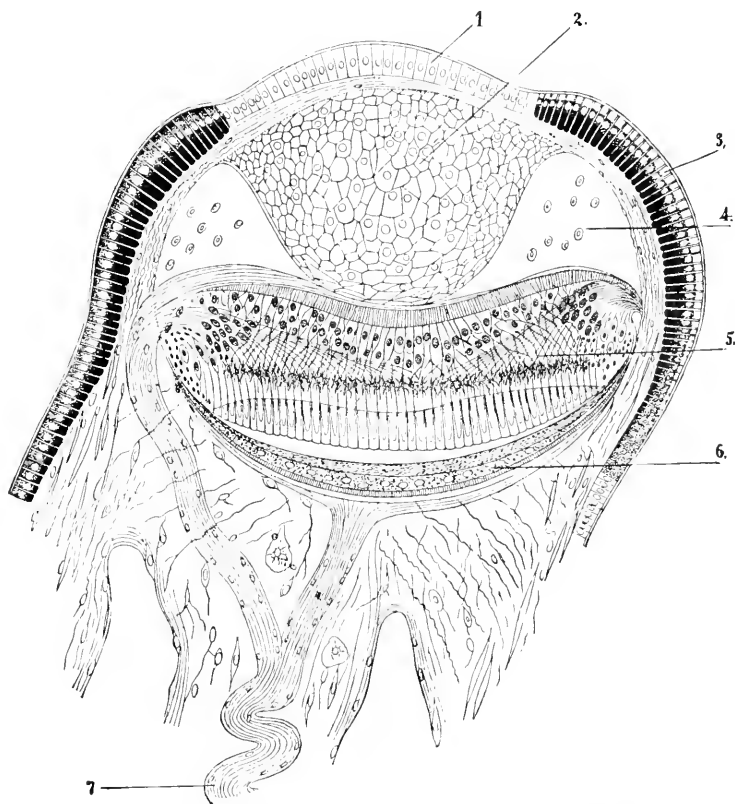
Fig. 151. Schnitt durch ein Mantelauge von Pecten. Nach W. PATTEN (1886), aus HATSCHER's Lehrbuch. 1 Epithel der Cornea. 2 Linse (soll nach PATTEN vom Bindegewebe der Cornea gebildet werden). 3 pigmentierte Epidermis in der Umgebung der Cornea (begrenzt die Pupille). 4 Blutsinus in der Umgebung der Linse. 5 Retina, bestehend von vorn nach hinten aus: innere Faserschicht, Ganglienzellenschicht, äußere Faserschicht, Sehzellen und Stäbchen. 6 Pigmentepithel, vor welchem das Tapetum. 7 Sehnerv, in 2 Aesten den Augenbecher umgreifend.
