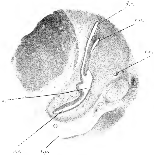
Fig. 114. Horizontalschnitt durch den Kopf eines Mäuseembryos von 13 Tagen. c.a. und c.c. vorderer und äußerer Bogengang. d.e. Ductus endolymphaticus. s. Sacculus. c.c. Canalis cochlearis. t.p. tubo-tympanaler Raum.
