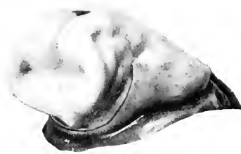
Fig 159. Rostralaterale Ansicht des Kopfendes eines Schweinsembryo ( Sus scrofa ), 4,7 mm Körperlänge, 10 Urvirbel, 16 Tage. Modell von KEIBEL (1897). Vergr. ca. 25:1.
