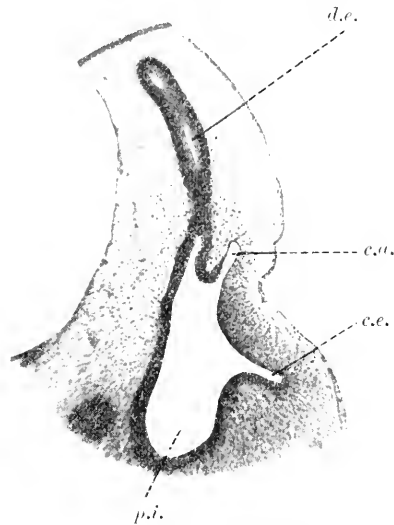
Fig. 113. Horizontalschnitt durch die Labyrinthblase eines Embryos von Scyllium canic . d.e. Ductus endolymphaticus, c.a. und c.e. vordere und äußere Bogengangstasche. p.i. Pars inferior-labyrinths.
