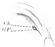
Fig. 27. Salamandra maculata in der Metamorphose. Gaumenfläche. Vergr. 7:1. Nach SEYDEL (1895). Ch Choane, GP Gaumenfortsatz.
