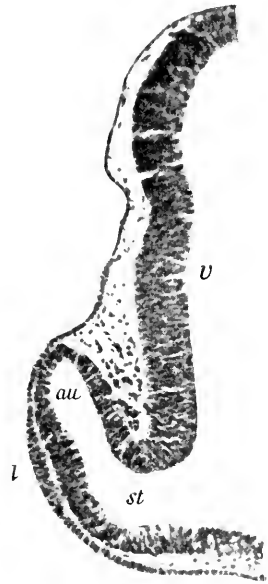
Fig. 177. Schnitt durch den Vorderkopf eines Embryo von Torpedo ocellata von 5,4 mm. Präp. von A. FROEYER. Vergr. 100:1. au Sehventrikel in der Augenblase. l Linsenplatte des Ektoderms. st Stiel der Augenblase. v Ventrikel im Zwischen- und Mittelhirn.
