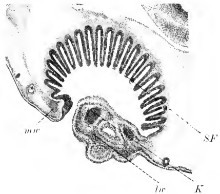
Fig. 14. Schnitt durch das Geruchsorgan eines Acanthias-Embryos von 47 mm Länge. Vergr. 50:1. Nach BERLINER (1902). K Knorpel. mw medialer, lr lateraler Wulst. SF SCHNEIDER'sche Falten.
