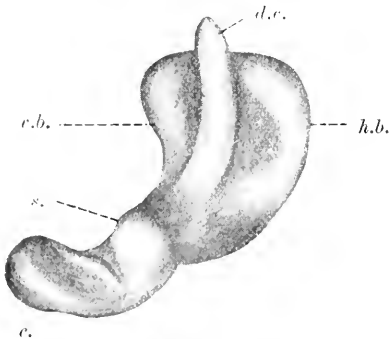
Fig. 108. Modell des Labyrinths eines Schweineembryos von 18 mm N.St.L. Medialansicht. c.b. und h.b. vorderer und hinterer Bogengang. d.e. Ductus endolymphaticus. s. Sacculus. s. Schnecke.
