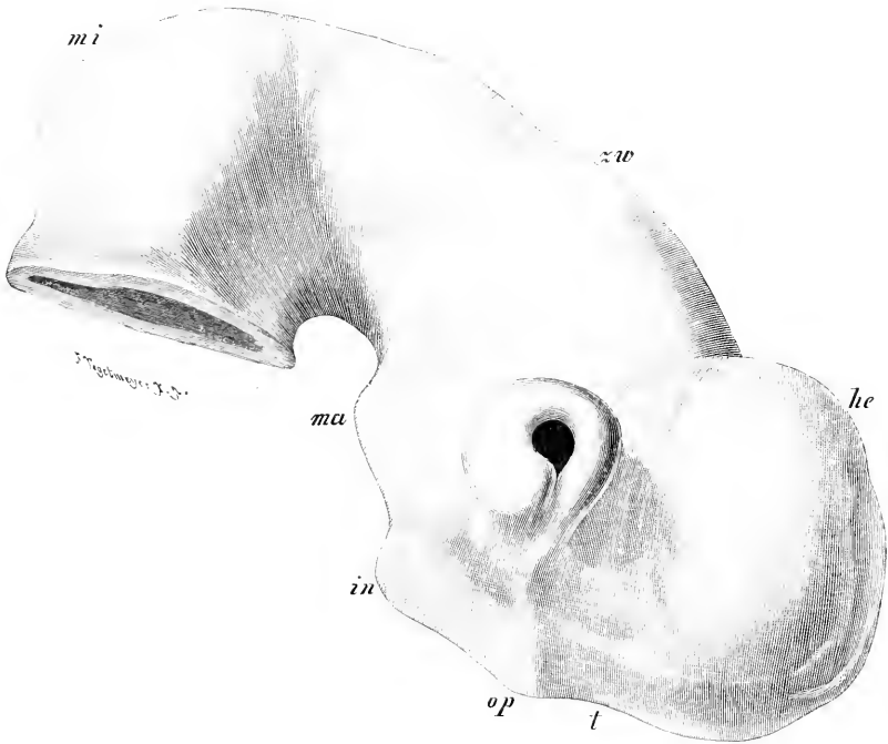
Fig. 188. Mittel- und Vorderhirn eines menschlichen Embryo von Ende der 1. Woche, Ansicht von rechts und unten. Mit Benutzung des Modells von HIS und ZIEGLER, Serie XXII, No. 1. Vergr. ca. 37 : 1. he Hemisphärenblase. in Trichter. ma Proc. mamillaris. mi Mittelhirn. op Torus opticus. t Lamina terminalis. zw Zwischenhirn.
