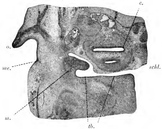
Fig. 140. Horizontalschnitt durch den Kopf eines 14 Tage alten Mausembryos. schl. Rachenhöhle. th. tubo-tympanaler Raum. m. Anlage des Hammers. mc. Anlage des äußeren Gehörganges. o. Ohrmuschel. c. Schnecke.
