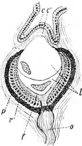
Fig. 150. Schematischer Durchschnitt durch ein Rückenauge von Onchidium . Nach C. SEMPER (1877). c und c' Epithel und Bindegewebe der Cornea. l Linse, bestehend aus sehr großen Zellen, die den Augenbecher ganz ausfüllen. o Sehnerv. f , r , p Nervenfaserschicht, Stäbchenzellen- und Pigmentschicht der Retina.
