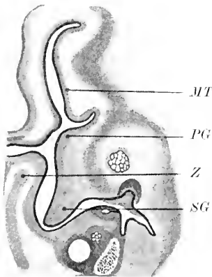
Fig. 64. Frontalschnitt durch die Nasengegend eines Rindsembryos. Nach DURSUY (1869). MT Maxilloturbinale. PG primitive, SG sekundäre Gaumenleiste. Z Zunge.
