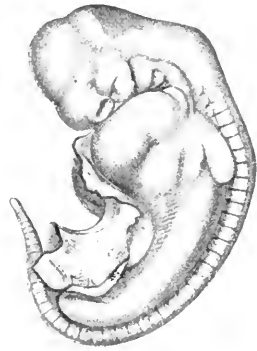
Fig. 59. Schweins-embryo von 20 Tagen mit Nasengrube. Vergr. 5:1. Nach KEIBEL (A. L. II. 1897).
