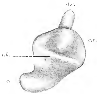
Fig. 88. Modell der Hörblase eines Kaninchenembryos von 8 mm N.St.L. Lateralansicht. d.e. Ductus endolymphaticus. t.v. Tasche für die vertikalen Bogengänge. t.h. Tasche für den horizontalen Bogengang. c. Ductus cochlearis.
