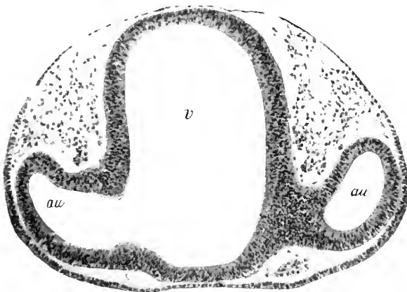
Fig. 166. Querschnitt durch den Vorderkopf eines Hühnerembryo aus dem letzten Drittel des 2. Brüttagcs. Präp. von M. HEIDENHAIN. Vergr. 100:1. au Schventrikel der Augenblase. v Ventrikel des Vorderhirns.
