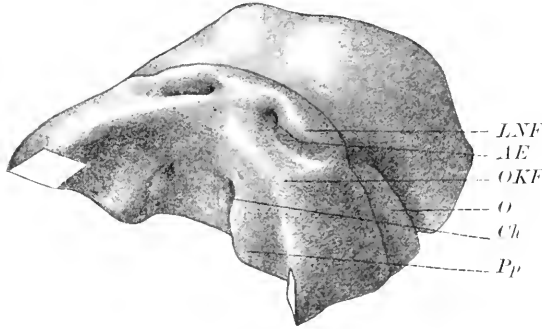
Fig. 62. Modell des Vorderkopfes eines menschlichen Embryos von 15 mm Länge. No. B anat.-biol. Inst. Berlin. Vergr. 12,5:1. AE Apert. externa. Ch primitive Choane. LNF lateraler Nasenfortsatz. O Auge. OKF Oberkieferfortsatz. Pp Processus palatini.
