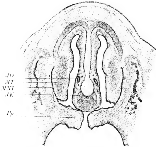
Fig. 65. Schnitt durch das Geruchsorgan eines menschlichen Embryos von 28 mm Länge. G. 33 anat.-biol. Inst. Berlin. Vergr. 20:1. JO JAKOBSON'sches Organ. JK JAKOBSON'scher Knorpel, MI Meatus narium inferior. MT Maxilloturbinate. Pp Processus palatini.
