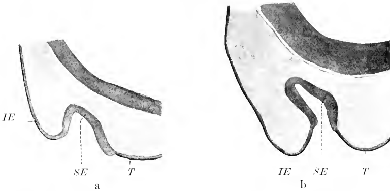
Fig. 39a und b. Schnitt durch das Geruchsorgan von Hühnerembryonen von 4,1 und 6,0 mm Kopfgröße. SE Sinnesepithel. IE indifferentes Epithel. T Teloderm.
