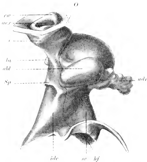
Fig. 32. Rana fusca von 31 mm Länge. Modell des rechten Geruchsackes von der Kopfspitze gesehen. Nach HINSBERG (1901). acr Apert. externa, c Einführungsgang, lf Choanenfalte, ide indifferentes, se Sinnesepithel, la lateraler Appendix, O Oberhaut, vr Ringwulst, sp Sporn, abl unterer Blindsack, idr untere Drüse.
