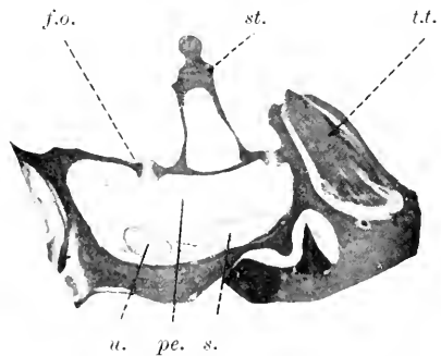
Fig. 133. Schnitt durch das Gehörorgan des Meerschweinchens. u. Utriculus. s. Sacculus mit seiner Macula acustica. pe. Cisterna perilymphatica. st. Stapes. f.o. Rand des Foramen ovale. tt. Musculus tensor tympani.
