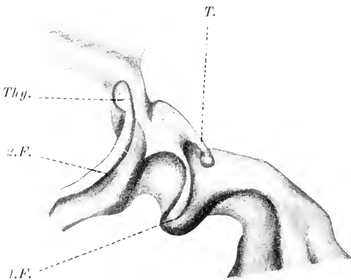
Fig. 137. Modell der Schlundhöhle einer 5 mm langen Froschlurve (nach SPEMANN 1898). 1.F. , 2.F. erste und zweite Schlundfalte. T. Tube. Th.y. Thymus.
