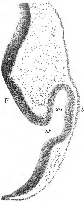
Fig. 167. Horizontalschnitt durch den Vorderkopf eines Hühnerembryo vom Ende des 2. Brütages. Präp. von M. HEIDENHAIN. Vergr. 100:1. au Schventrikel der Augenblase. l Linsenplatte des Ektoderms (oberer Rand). st Stiel der Augenblase. v Ventrikel des Vorderhirns.
