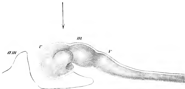
Fig. 165. Linksseitige Profilansicht des Gehirns von einem Hühnerembryo aus dem letzten Drittel des 2. Brüttagcs. Vergr. 40:1. am Kopfkappe des Amnion, m Mittelhirn, r Rautenhirn, v Vorderhirn. Der Pfeil bezeichnet die Lage des in Fig. 164 abgebildeten Schnittes.
