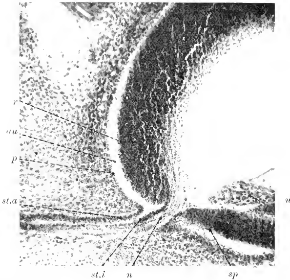
Fig. 235. Querschnitt des Auges einer Torpedo ocellata von 21 mm Länge. Präp. von M. FRORIEP. Vergr. 100:1. au Rest des Schventrikels. n Sehnervenfasern. p Pigmentblatt. r Retinalblatt. sp Ventral-rostrale Lippe der Becherspalte. st.a äußere, st.i innere Wand des Augenblasenstiels. w Wulst in der Spaltennaht, schräg geschnitten.
