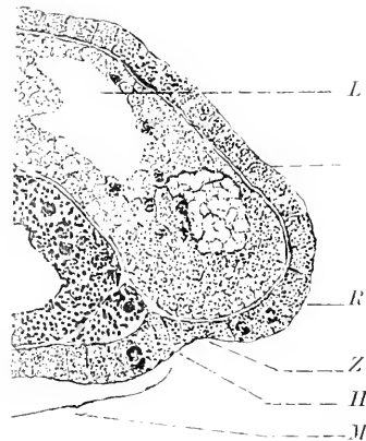
Fig. 3. Medianschnitt durch den Kopf eines 10 Tage alten Ammocoetes. Vergr. 150:1. Nach LUBOSCH (1901). R Riechplatte. II Hypophysenanlage. M Mundplatte. L Gehirnlumen. Z Zwischenplatte.
