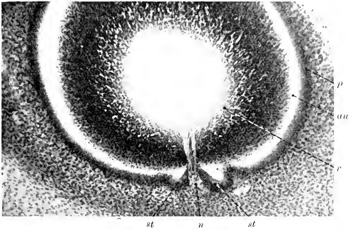
Fig. 236. Sagittalschnitt durch den Vorderkopf eines Embryo von Anas domestica , 122 Stunden bebrütet. Präp. von H. GRÖNROOS. au Sehgrube = Höhle der Augenblase, Sehventrikel. n Sehnervenfasern. p Pigmentblatt des Augenbechers. r Retinalblatt des Augenbechers. st Stiel der Augenblase.
