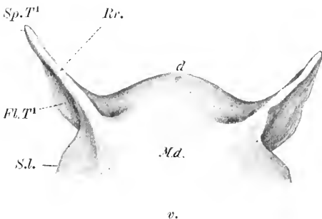
Fig. 139. Modell der hinteren Hälfte der Mundrachenhöhle eines 13 Tage alten Kaninchenembryos (nach PIERSOL 1888). Sp.T 1 , Fl.T 1 Spitze, Flügel der ersten Schlundtasche. s.l. Sulcus lingualis. Rr. Rachenrinne, d. dorsale, v. ventrale. Md. Dach der Mundrachenhöhle.
