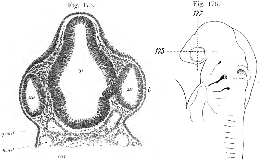
Fig. 175. Querschnitt durch den Kopf eines Embryo von Torpedo ocellata von 5,8 mm. Präp. von A. FRORIEP. Vergr. 100:1. au Augenblase, car Querkommissur der Carotis interna. l Ektoderm am oberen Rand der Linsenplatte. mnd mandibulare, pmd prämandibulare Kopfhöhle. v Zwischenhirn.
