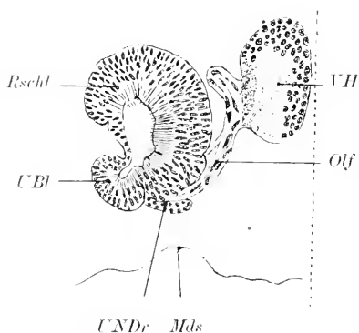
Fig. 26. Triton alpestris , 18 mm, Larve, Geruchssack. Querschnitt. Vergröß. 60:1. Nach BURCKHARDT (1891). Mds Mundschleimhaut. Olf Olfactorius. Rschl Riechschleimhaut. UBl unterer Blindsack. UNDr untere Nasendrüse. VII Vorderhirn.
