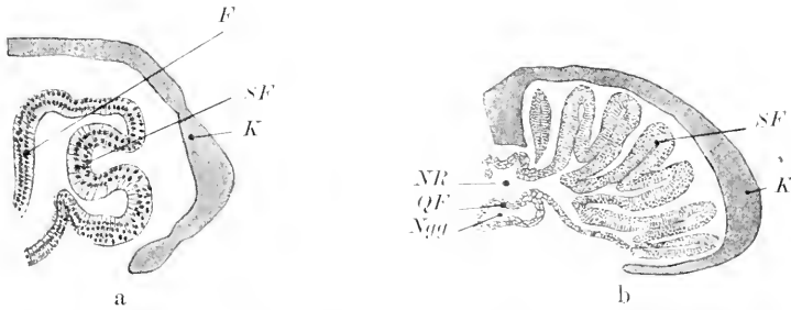
Fig. 7. Querschnitte durch die rechte Seite der Nasenhöhle von Ammocoetes am Beginn (a), und Ende (b) der Metamorphose. Nach KAENSCHKE (1889). K Knorpelkapsel. MF Mittelfalte. Xgg Nasengaumengang. NR Nasenrohr. QF Querfalte im Nasenrohr. SF seitliche Falten.
