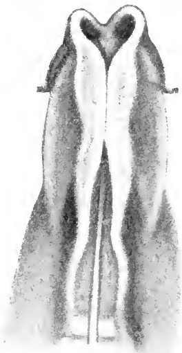
Fig. 153. Dorsalansicht eines Hühnerembryo vom Anfange des 2. Tages bei auffallendem Licht. Nach E. DURSÝ (1869).
