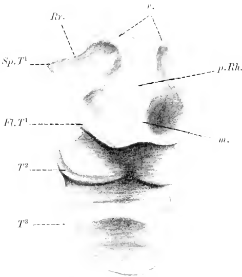
Fig. 136. Modell des Schlundspaltengebietes eines Kaninchembryos von 9 Tagen 11 Stunden (nach PIERSOL 1888). v. vordere seitliche Vertiefung der Rachenhöhle. Rr. Rachenrinne. Fl.T 1 , Sp.T 1 Flügel und Spitze der ersten Schlundtasche. p.Rh. primäre Rachenhöhle. m. Ausbuchtung zwischen den inneren Enden des ersten Bogenpaares. T 2 , T 3 zweite und dritte Schlundtasche.
