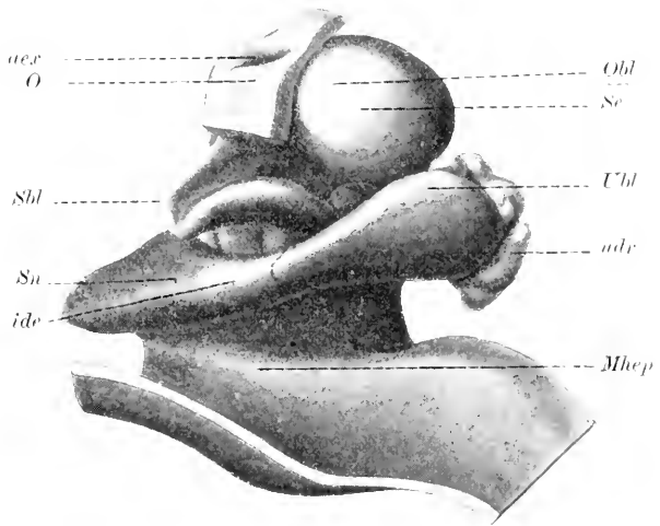
Fig. 33. Rana fusca in Metamorphose; rechter Geruchssack. Nach HINSBERG (1901). Ansicht von der Kopfspitze. Mhsp Mundhöhlenepithel. Obl oberer Blindsack. Sbl seitlicher Blindsack. Su seitliche Nasenrinne. Uebrigere Bezeichnungen wie in Fig. 32.
