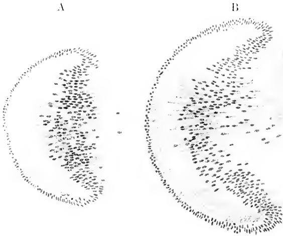
Fig. 210. Linsenentwicklung von Lepus cuniculus . Fortsetzung zu Fig. 209. Nach RABL. Vergr. 93:1. Alter der Embryonen: A 14 Tage, B 15 Tage.
