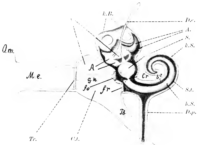
Fig. 76. Schematische Darstellung des menschlichen Gehörorgans nach WIEDERSHEIM. A. Ampullen. Cr. Canalis reuniens. Ct. Paukenhöhle. D.e. Ductus endolymphaticus. F.o. Foramen ovale. F.r. Foramen rotundum. G.k. Gehörknöchelchen. h.B. häutige Bogengänge. h.S. häutige Schnecke. k.B. knöcherne Bogengänge. k.S. knöcherne Schnecke. M.e. äußerer Gehörgang. O.m. Ohrmuschel. S. Sacculus. S.e. Saccus endolymphaticus. S.t. Scala tympani. S.v. Scala vestibuli. Tb. Tuba. Tr. Trommelfell. U. Utriculus. x Vorhofsblindsack. D.p. Ductus perilymphaticus.
