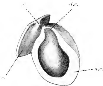
Fig. 82. Modell des Hörbläschens eines Kaninchenembryos kurz vor der Abschnürung; bei x die Abschnürungsstelle von der Epidermis ( e. ), d.c. die Anlage des Ductus endolymphaticus. Bei d.v. erscheint die Wand des Bläschens verdickt. Das ursprüngliche Modell ist halbiert.
