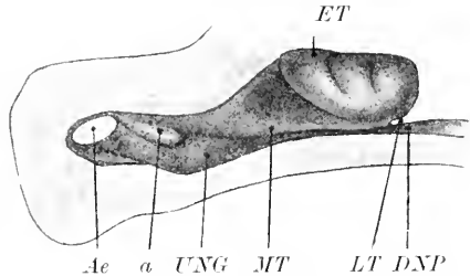
Fig. 71. Modell der lateralen Nasenwand eines Beuteltungen von Echidna (Std. 47, SEMON). Vergr. 20:1. Nach SEYDEL (1899). AE Apertura externa. ET Ethmoturbinalia. DNP Ductus nasopharyngeus. MT Maxilloturbinalia mit vorderem Wulste a . LT Lamina terminalis. UNG Unterer Nasengang.
