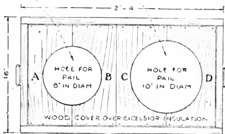
FIG. 149. — Plan.
