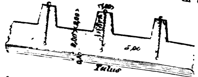
Fig. 1. Revêtement mit trapezförmigen Strebepfeilern.
