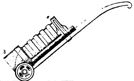
Fig. 3. Geschosskarre. a. Bügel zum Überklappen- Höher Holzklott.
