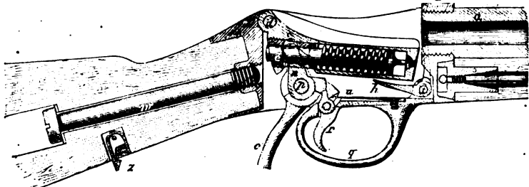
Fig. 3. Geöffnet mit zusammengepresster Spiralfeder.
