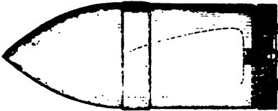
Palliser-Granate mit Gas-check.
