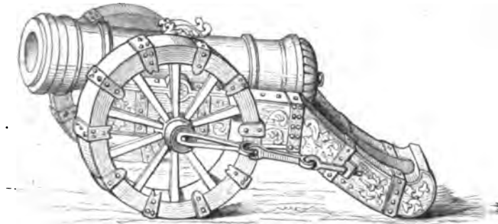
Fig. 3. Obusier (Feueckatze) de 1580. Rohr 6' lang Kaliber 6—10". Aus Napoleon „l'avenant" nach Semftenberg, Zeugmeister in Danzig.
