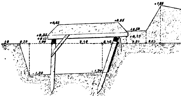
Hangard in einem Feldwerke.
