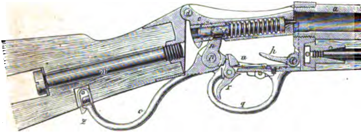
Fig. 2. Geschlossen mit loser Spiralfeder.
