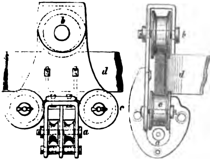
Fig. 4. Geschoss- oder Laufkatze. a. Talje zum Heben der Geschosse. b. Oberes Laufrad. c. Friktionsrader. d. Transportschienen.
