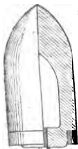
Granate mit Expansionsring nach Batters für die 30-lige Artillerie Rodman-Kanone.
