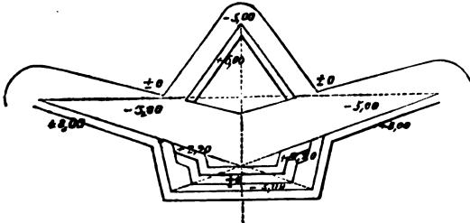
Verstärkte Grabenschere.
