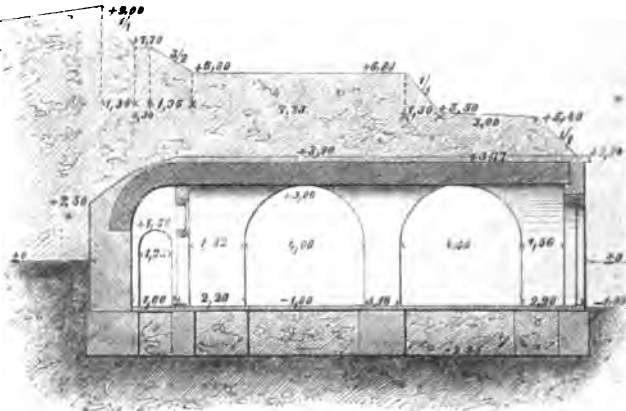
B. Profil.
