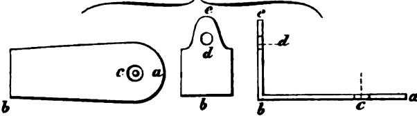
Fig. 7. Kolbenblech.
