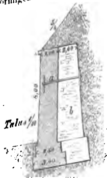
Fig. 3. Revêtement en surplomb. a. Anker. b. Strebe Pfeiler.
