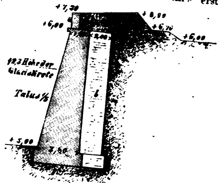
Fig. 2. Ganzes Eskarpen-Revêtement. a. Tabletmauer. b. Strebepfeiler.
