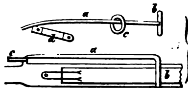
Fig. 10. Karabinerstange.
