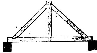
Einfaches Hängewerk.
