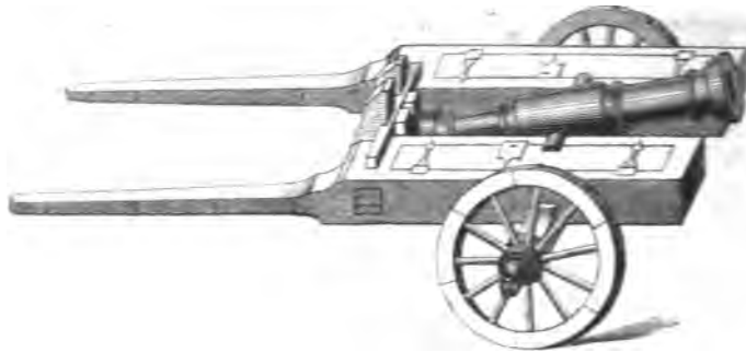
Karrenbüchse 1479—1480, Germ. Mus.
