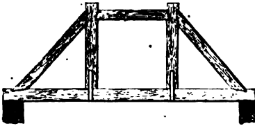
Doppeltes Hängewerk.
