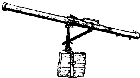
Raketongestell für den Gebrauch zur See.
