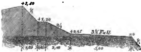
Profils des gedeckten Weges. (Ein Beispiel d. Grundrisses in der Skizze zum Artikel „Bastionär Tracé.“)
