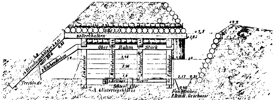
Bedeckte Batterie (Mörserstand versenkt erbaut. (Masse in m.)
