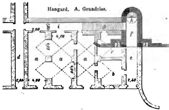
A. Hälfte des Grundrisses a. Mannschafterküche. b. Offiziersraum. c. Vorratsraum. d. Poterne zur Salilant-Kaponniere. e. Poterne für b, c und h. f. Hohltraverse auf dem Wallgange. g. Treppe von i nach f. h. Wendeltreppe von e nach f. i. Korridor. k. Nische für Geschosse in den Flügelmauern der Hohltraverse. Anmkg: Dunkle Schraffirung bedeutet im Grundriss: Mauerwerk über dem Wallgange; im Profil: Gewölbe.
