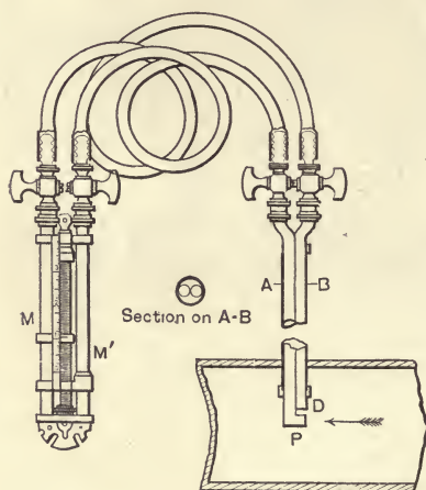
FIG. 18.—Pitot Tube.
