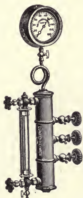
FIG. 166.—Water-column.
