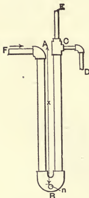
FIG. 175. Siphon-trap.
