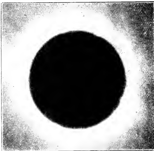
Wie eine Sonnenfinsternis aussieht. Bei einer Sonnenfinsternis geht der Mond zwischen der Erde und der Sonne hindurch.
