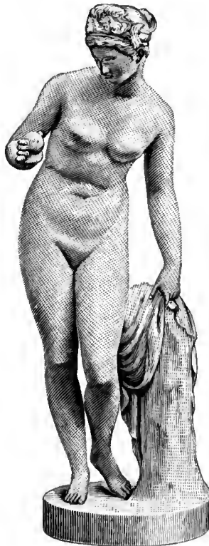
VENUS—THORWALDSEN.
