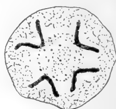
FIG. 6.—Same (polar view).
