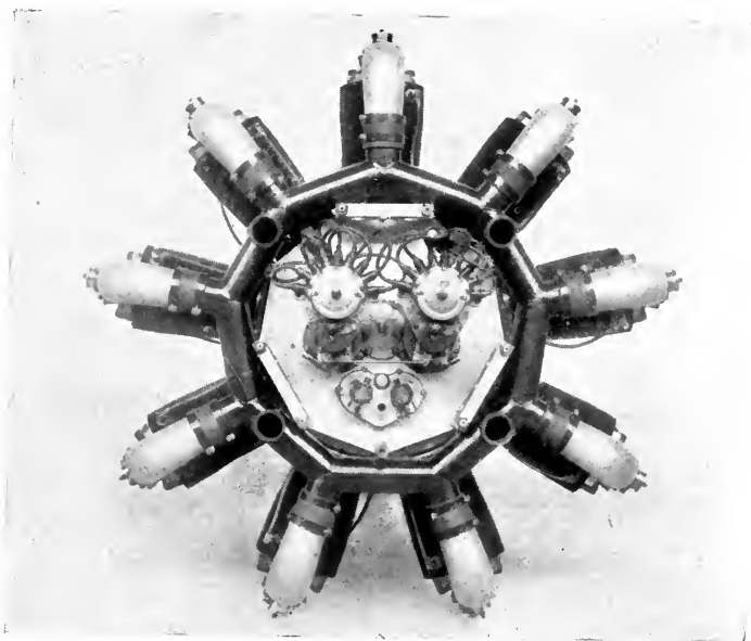
'Dragonfly' 1 A.
