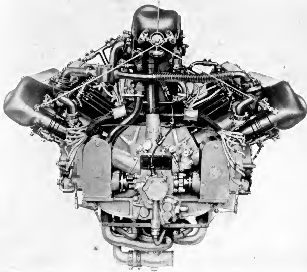
Napier 'Lion.'
