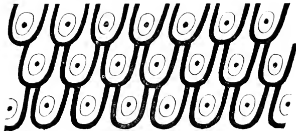
FIG. 150. SCALE-PATTERN (DAPHNAE).
