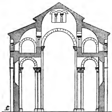
FIG. 97.—SECTION OF NOTRE DAME DU PORT, CLERMONT.
