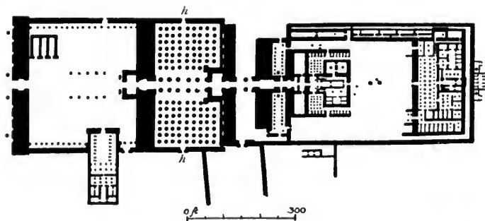
FIG. 11.—TEMPLE OF KARNAK. PLAN.
