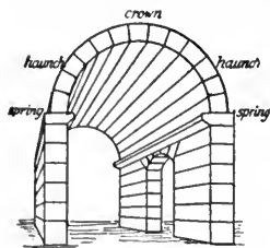
FIG. 46.—BARREL VAULT.
