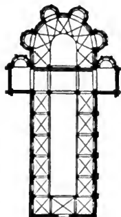
FIG. 96.—PLAN OF NOTRE DAME DU PORT, CLERMONT.
