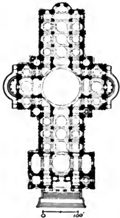
FIG. 186.—PLAN OF ST. PAUL'S, LONDON.
