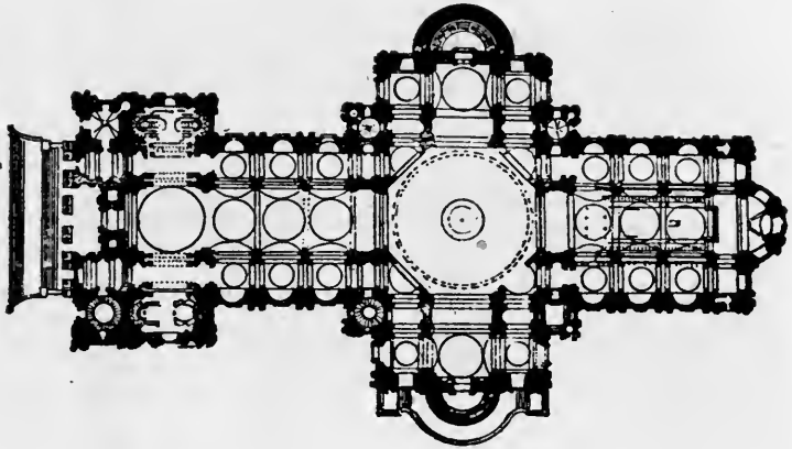
FIG. 244—LONDON. SAINT PAUL'S CATHEDRAL. PLAN
