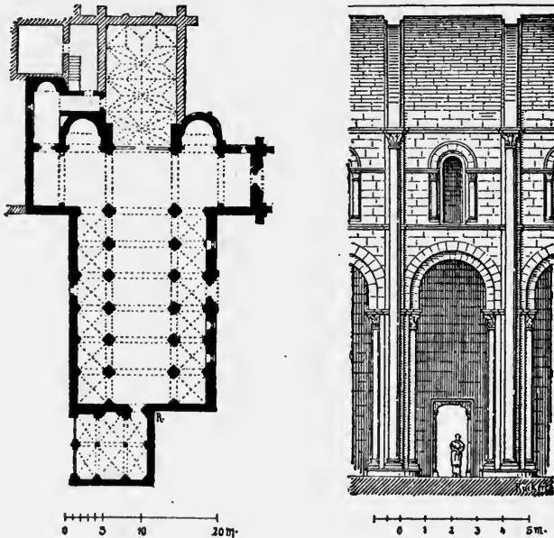
FIG. 136—LEON. SAN ISIDORO. PLAN AND SYSTEM
