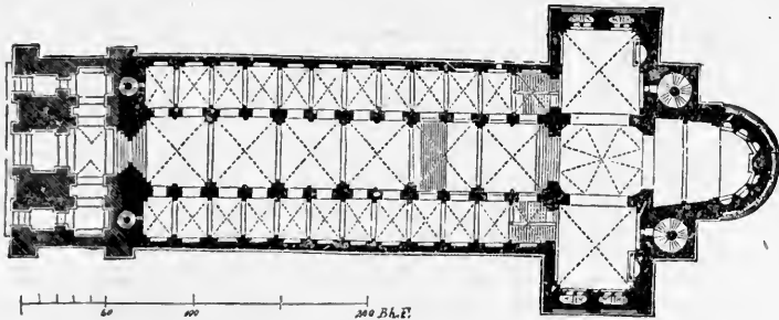
FIG. 115—SPEYER. PLAN
