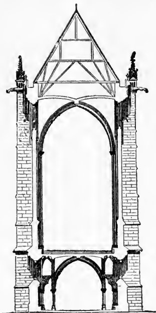
FIG. 148—PARIS. THE SAINTE CHAPELLE. TRANSVERSE CUT
