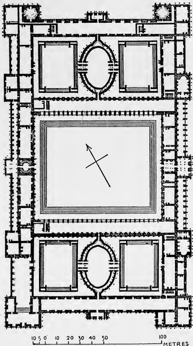
FIG. 214—PARIS. THE TUILERIES. (DE L'ORME'S PLAN)
