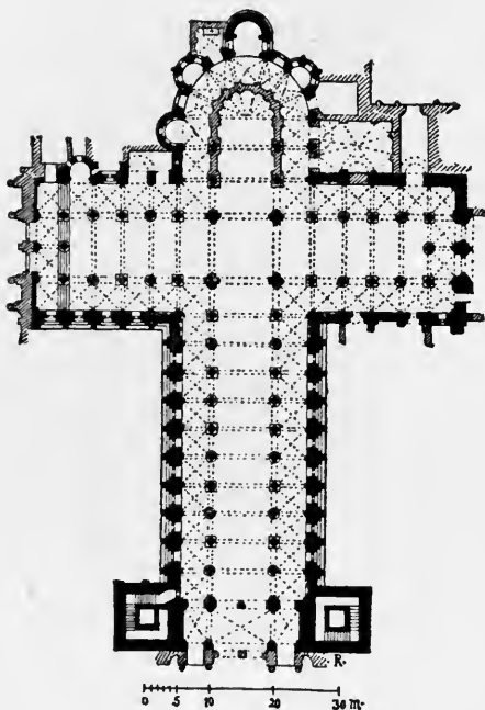
FIG. 135—COMPOSTELA. SANTIAGO. PLAN
