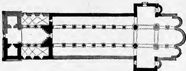
FIG. 112—PAULINZELLE. PLAN
