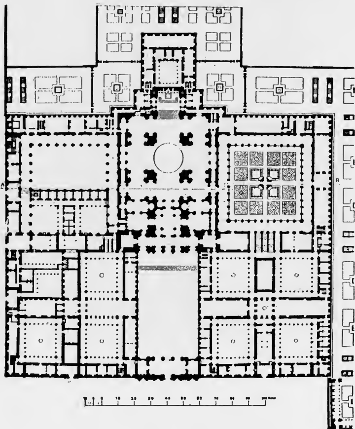
FIG. 231—THE ESCURIAL. PLAN
