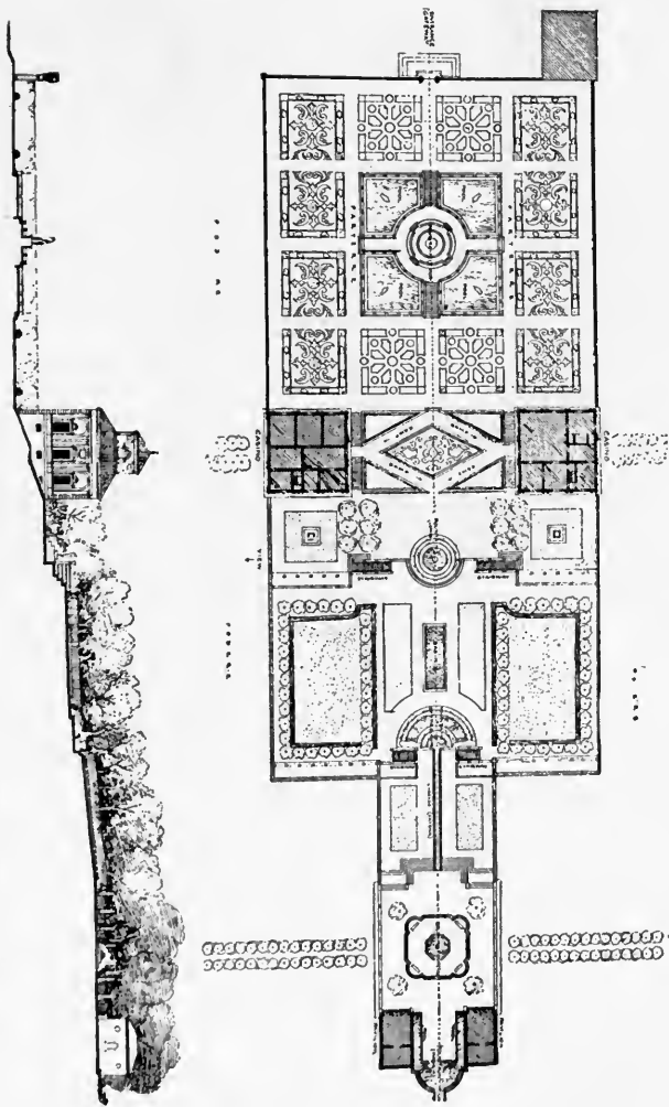
FIG. 230—BAGNAIA. VILLA LANTE. PLAN. (TRIGGS)
