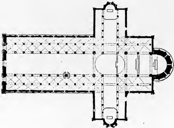
FIG. 106—PISA. CATHEDRAL. PLAN
