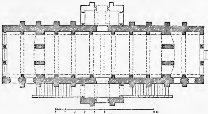
FIG. 98—SANTA MARIA DE NARANCO. PLAN
