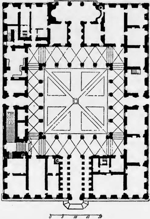
FIG. 209—ROME. PALAZZO FARNESE. PLAN
