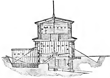
FIG. 3. SECTION ON A. B. (FIG. 1.)
