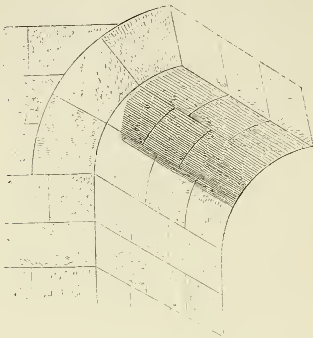
FIG. 78.—Arrangement of voussoirs.
