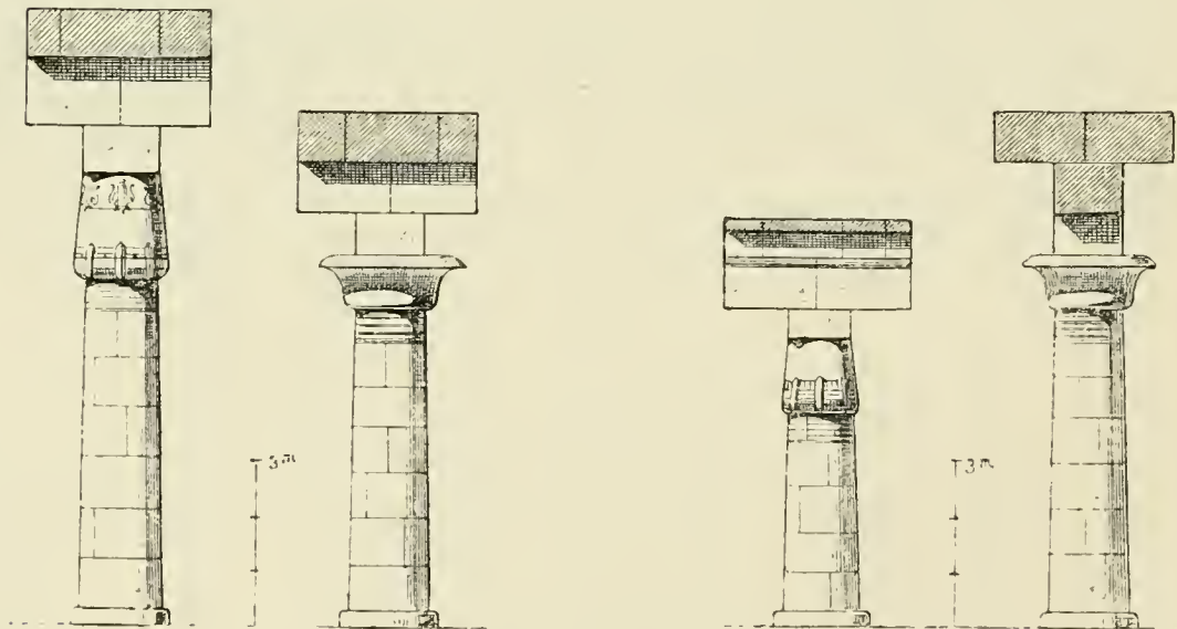
FIG. 63.—Temple of Khons, Thebes. ( Descr. de l'Égypte , t. iii., pl. 55.)
