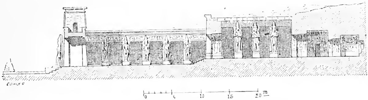
FIG. 239.—Gherf-Hossein, longitudinal section ; from Prisse.
