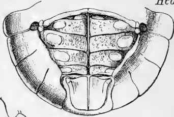
Pleon, ventral
