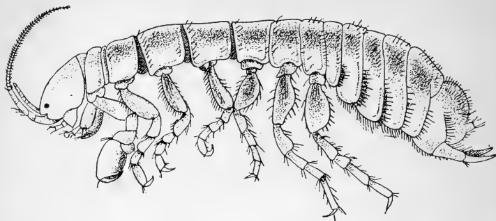
Phreatoicus australis
