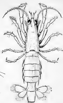
Upogebia littoralis
