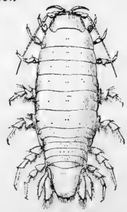
Cirolana borealis
