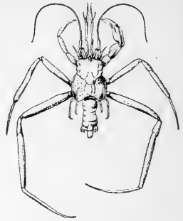
Tylasspis anomala
