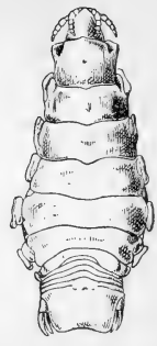
Ceratothoa auritus
