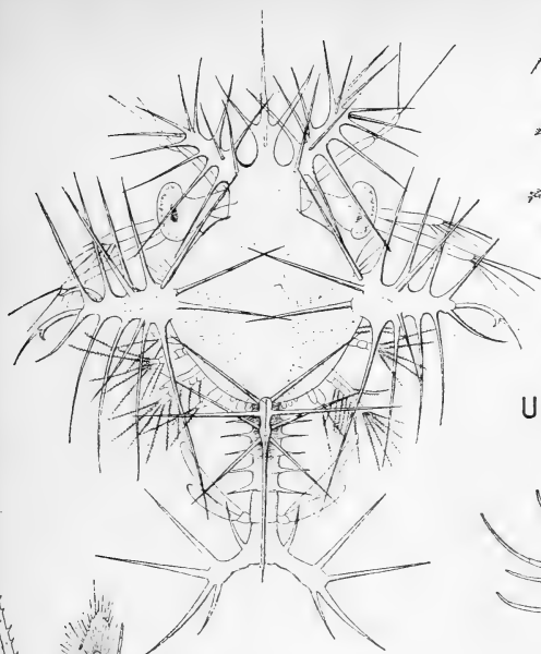
Elaphocaris Dohrni
