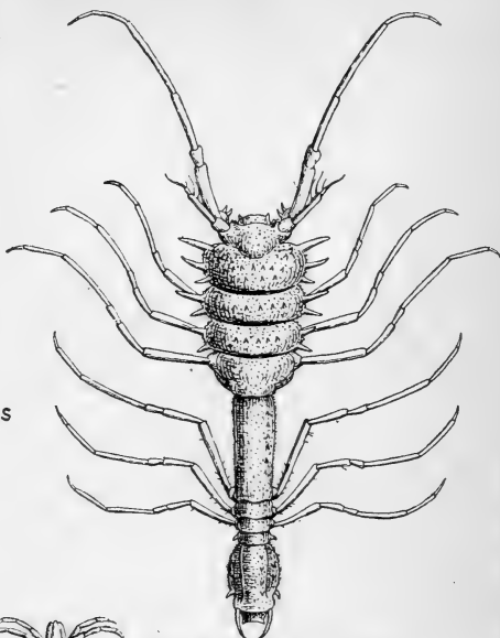
Ischnosoma spinosum
