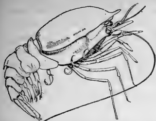
Notostomus perlatus
