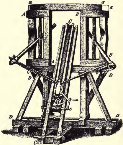
BALLISTA.
